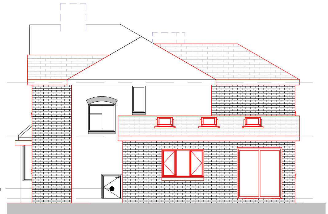
02-P-Elevation 1 : 100
