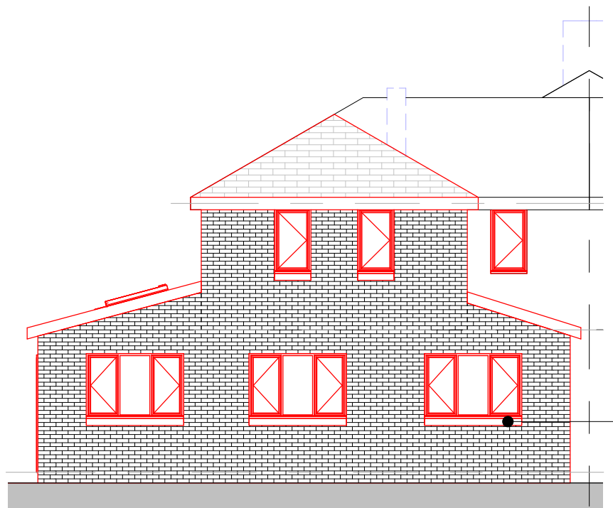
03-P-Elevation 1 : 100
