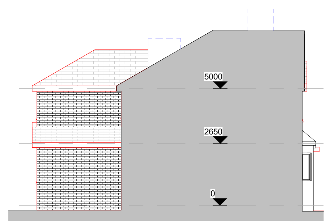
04-P-Elevation 1 : 100
