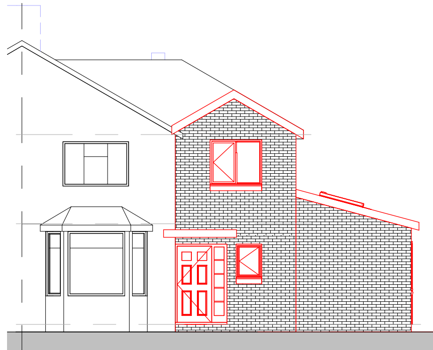
01-P-Elevation 1 : 100
