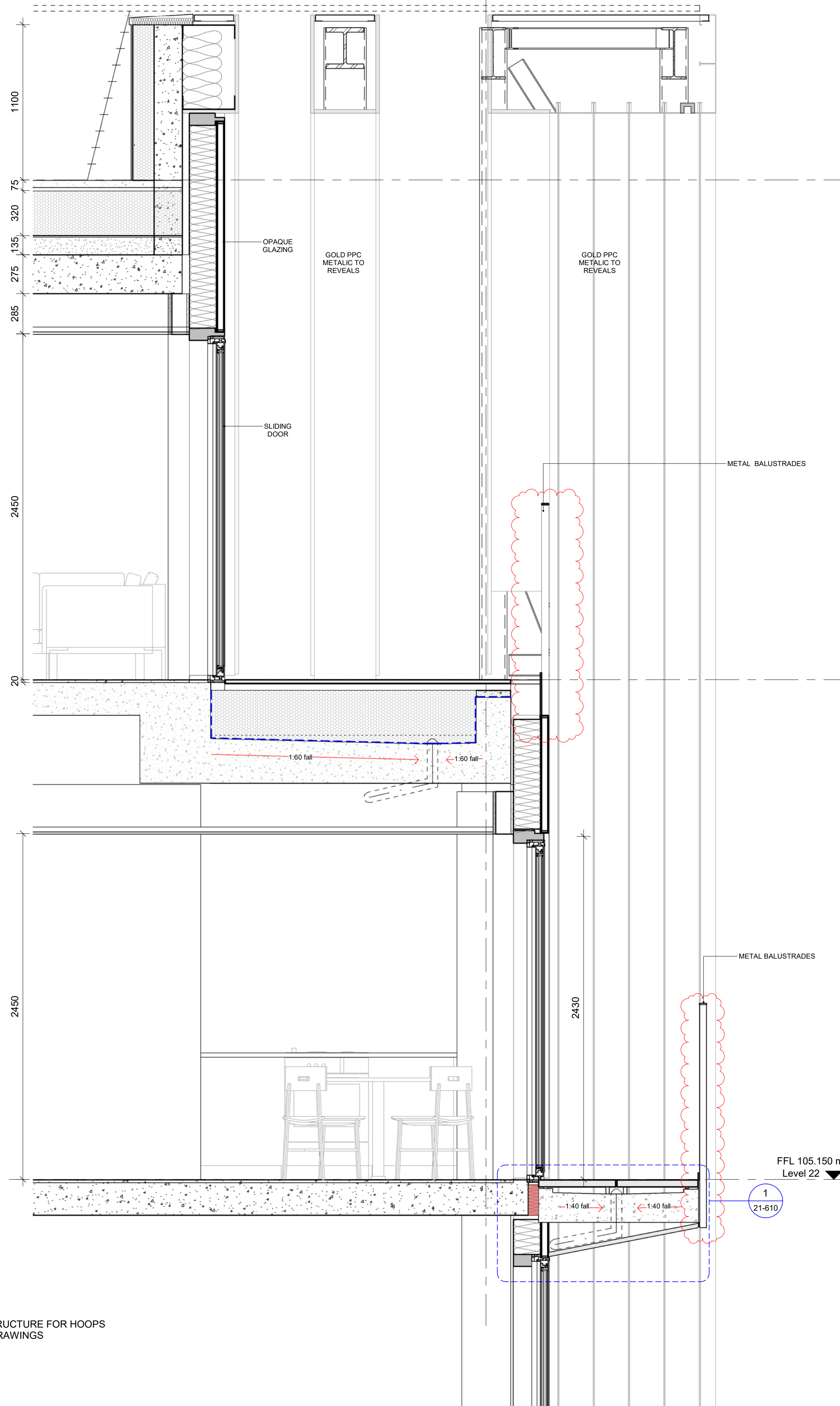
3 SECTION A 21-302 1 : 20
