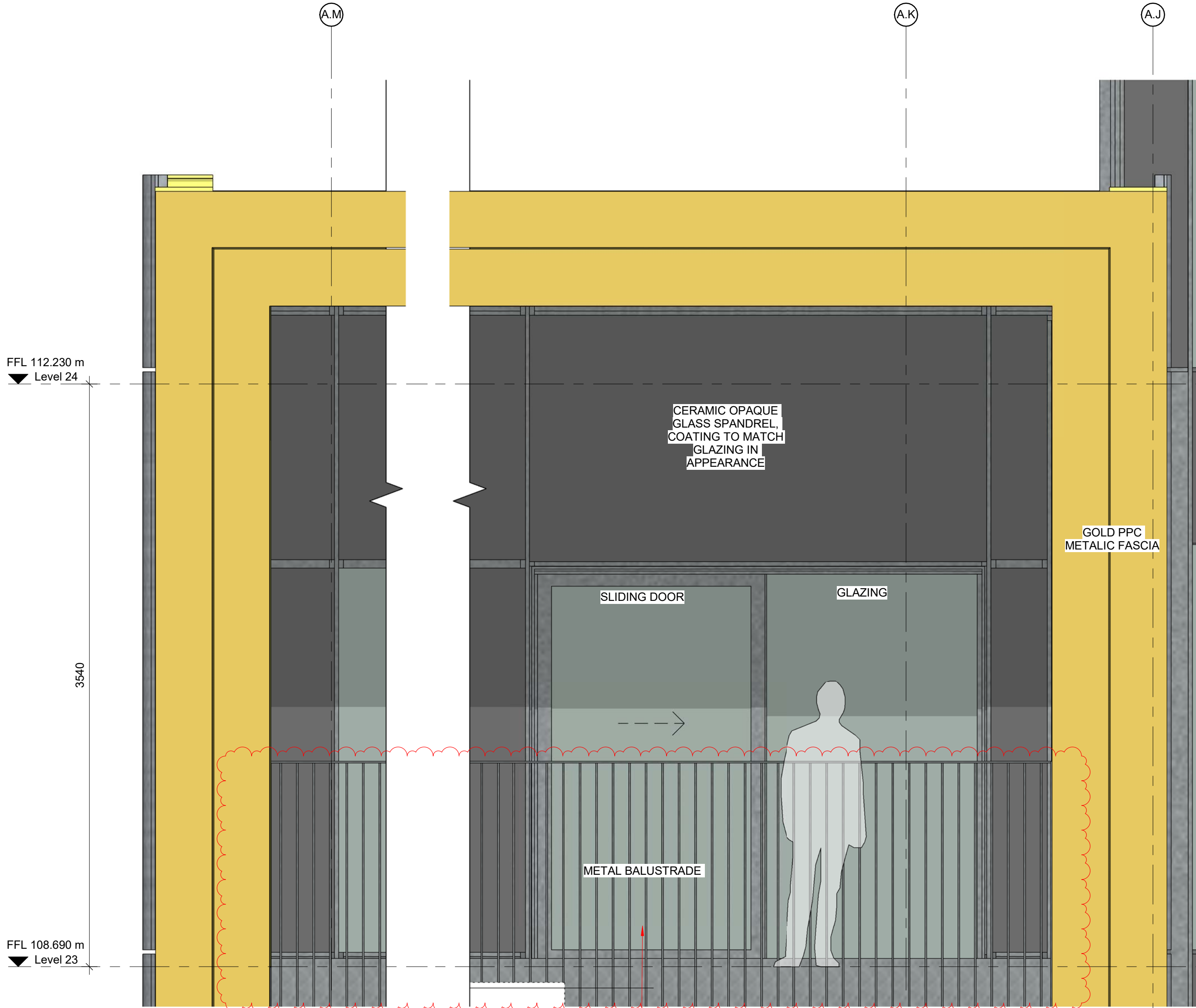
1 ELEVATION 20-411 1 : 20
