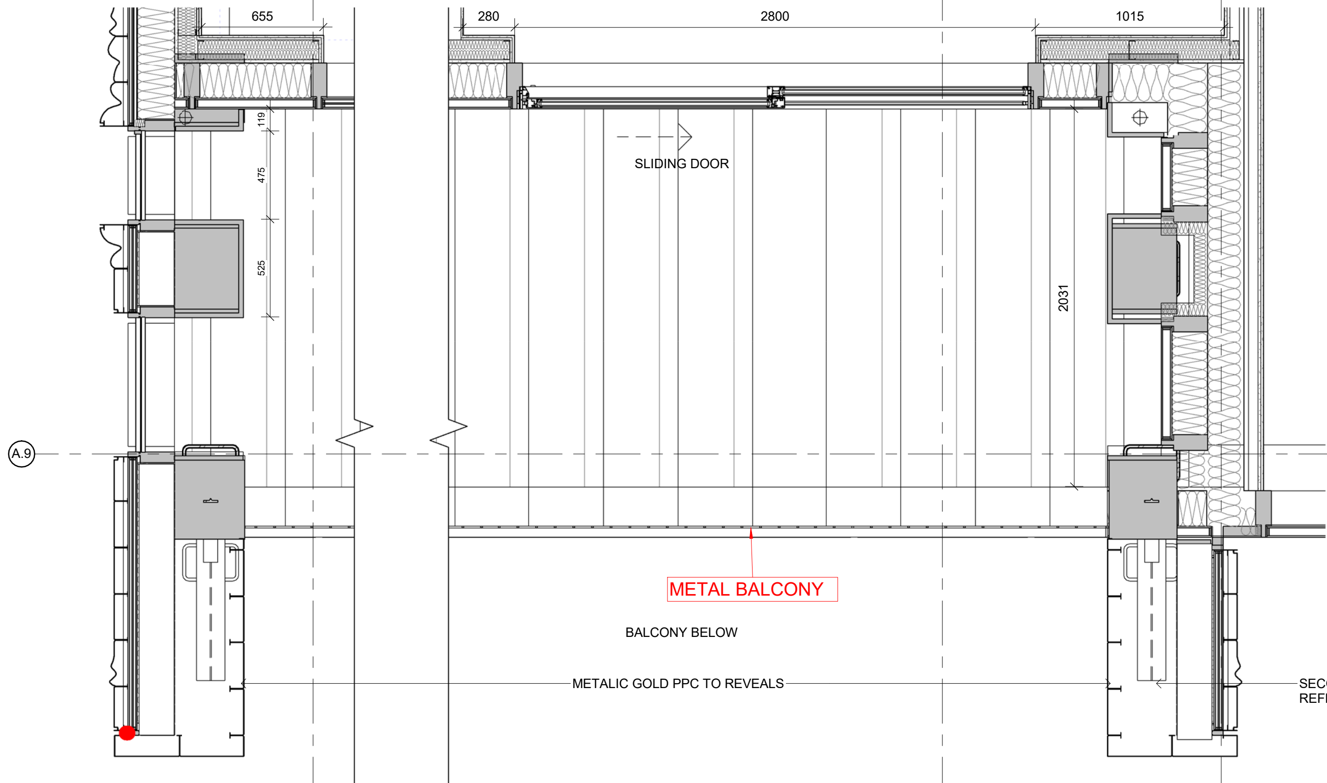
2 DETAIL PLAN 1 : 20
