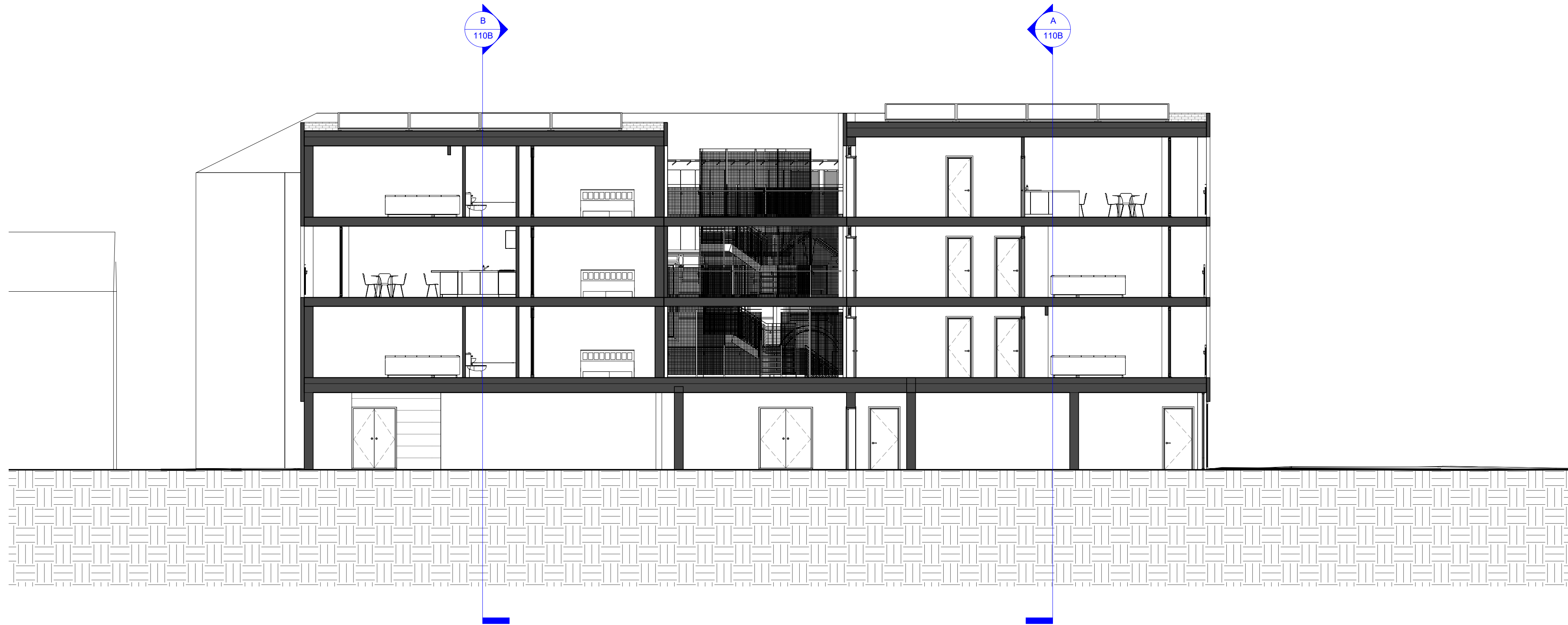
Section C 1 : 100
