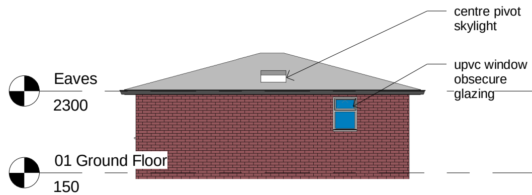
1 Right 1 : 100
