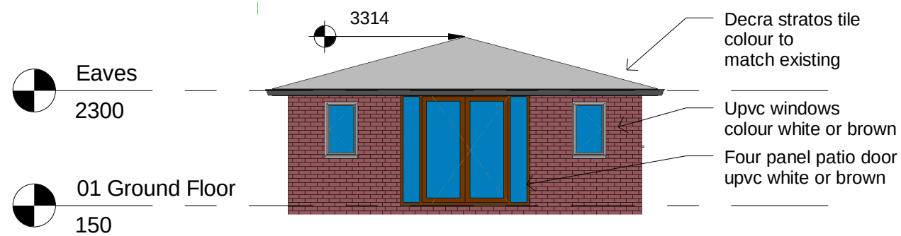
3 Front 1 : 100
