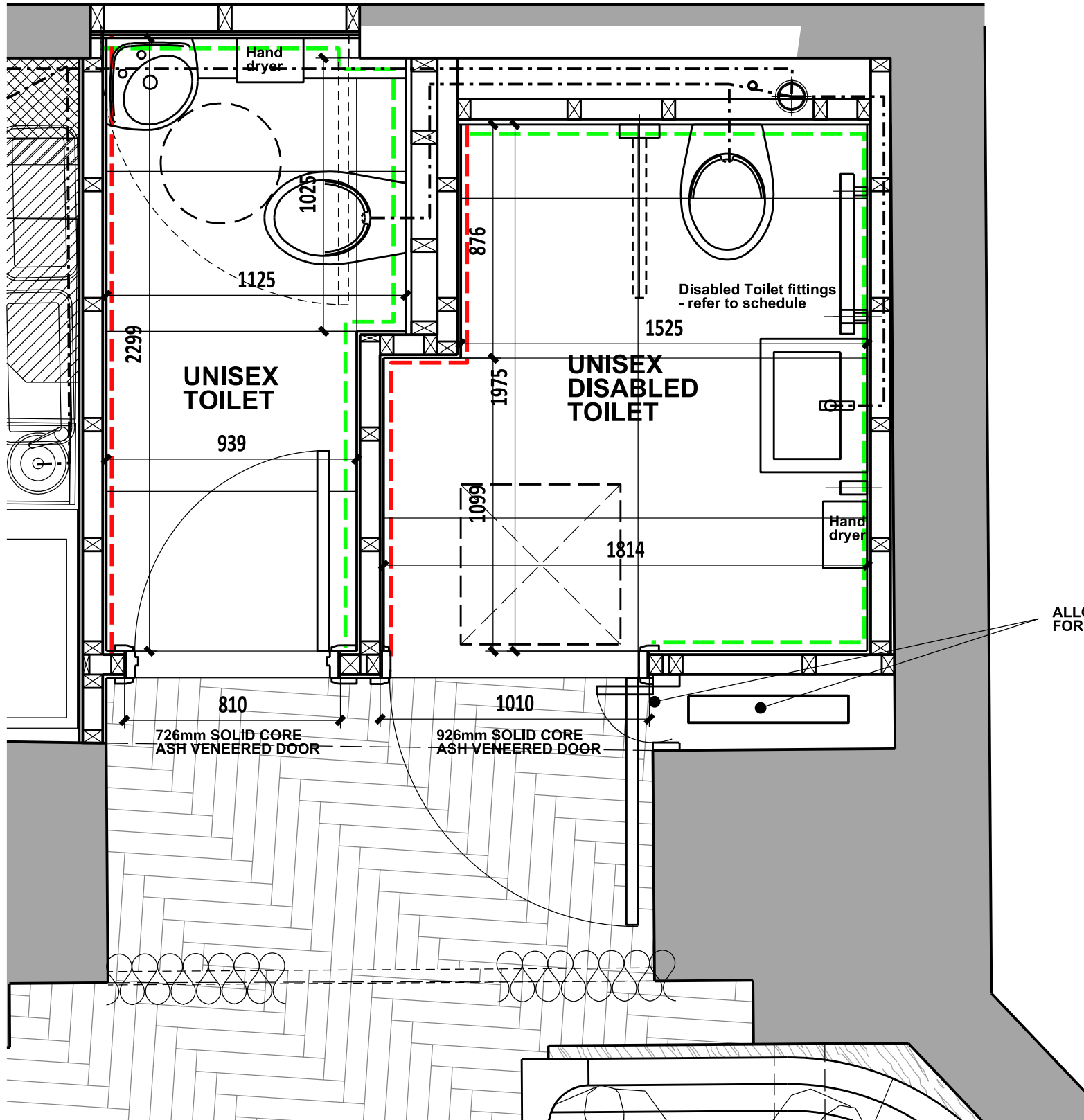
TOILET PLAN 1:20
