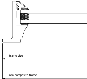
Section E - E
