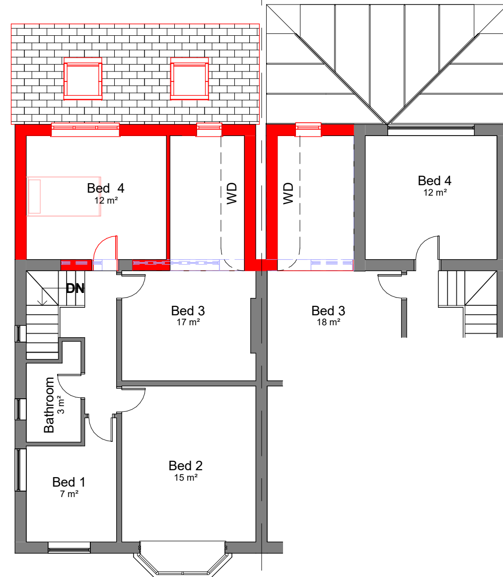
01-P-First Floor 1 : 100
