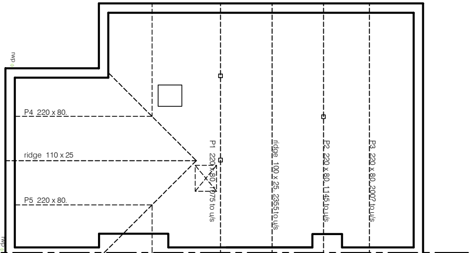
LOFT PLAN
