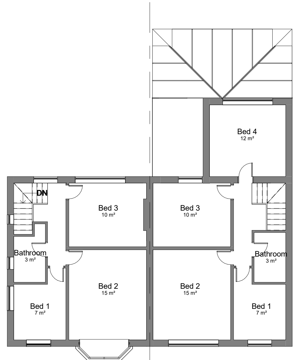
01-E-First Floor 1 : 100
