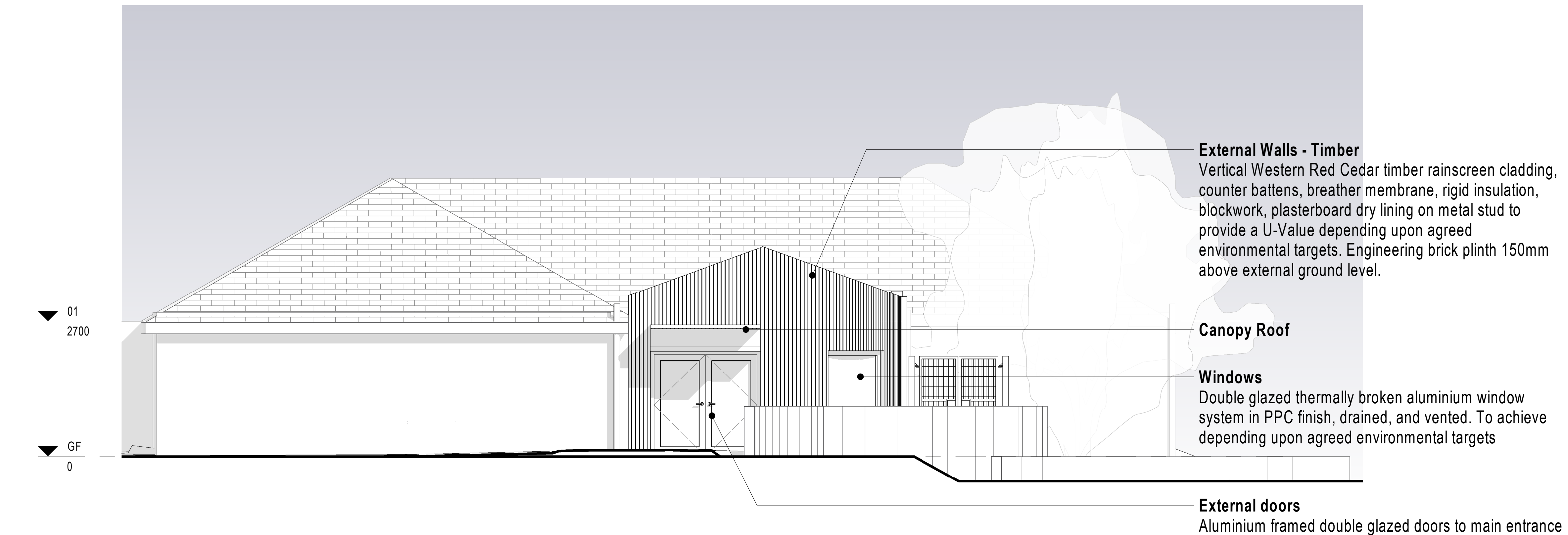
B Option 5 - Elevation B 1 : 50
