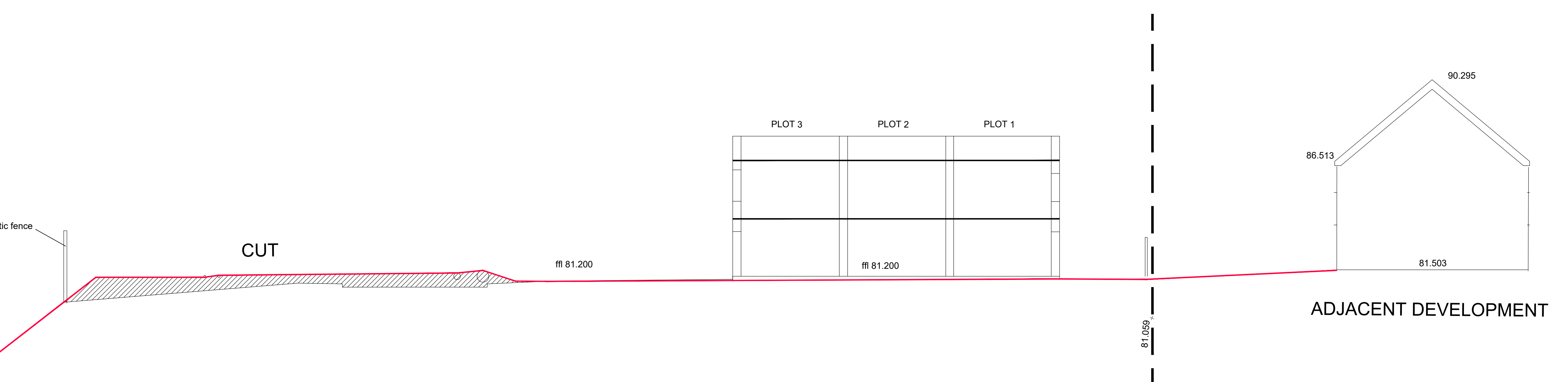
SECTION A-A
