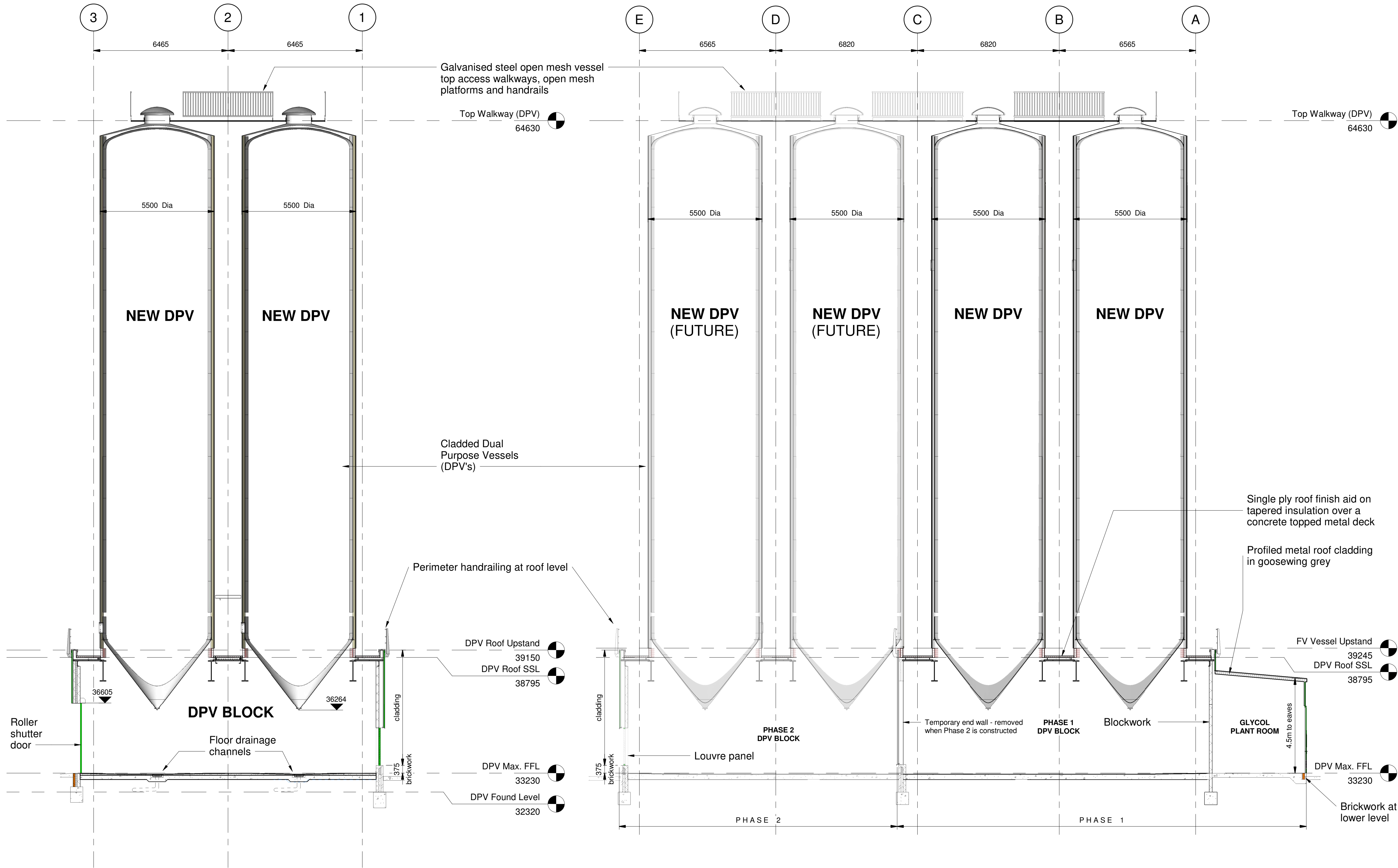
A DPV Block Section A-A 1 : 100
