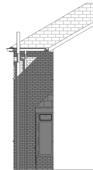
3 Side 1 : 100
