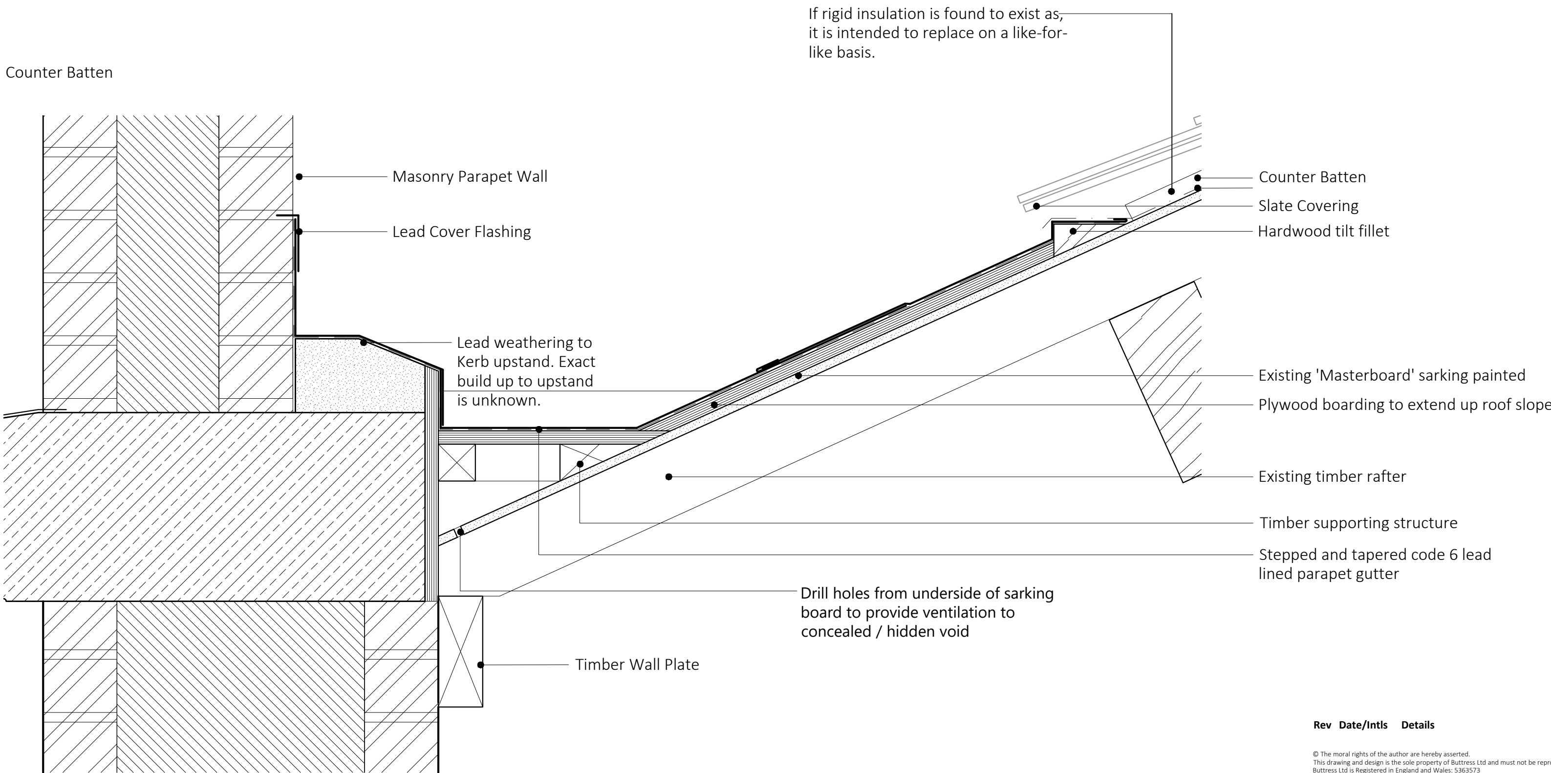
Detail A1 1:5
