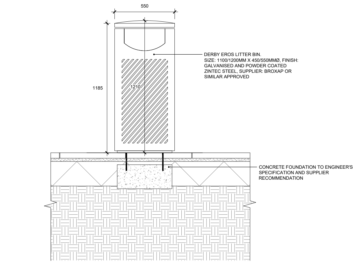
01A LITTER BIN 602 SECTION
