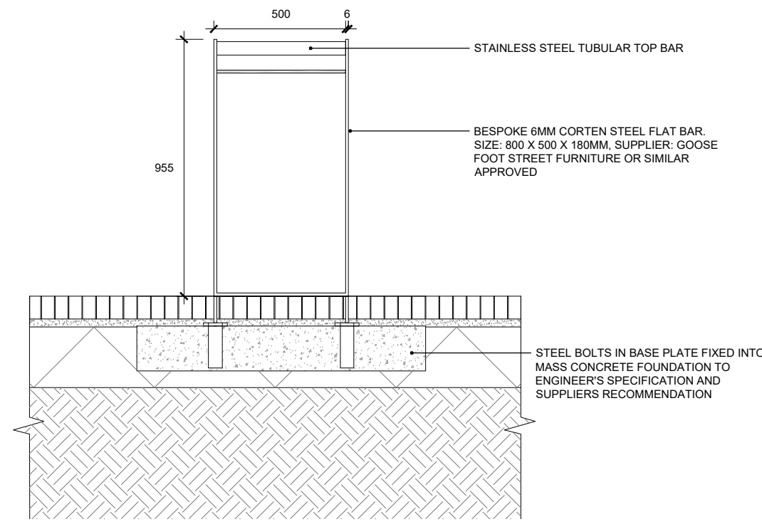
02A CYCLE STAND 602 PLAN
