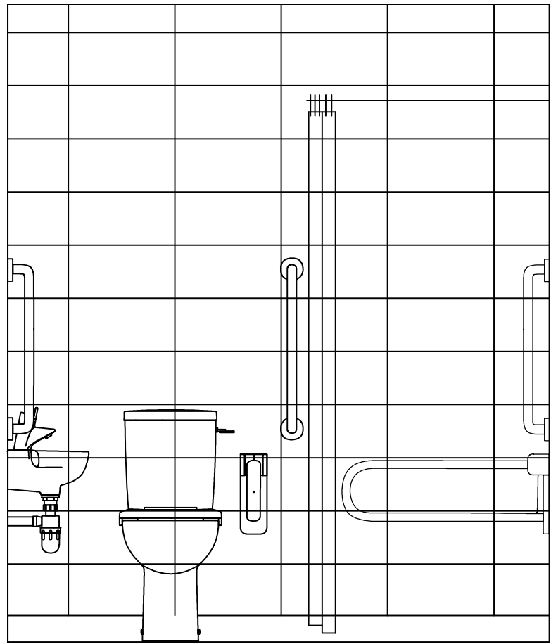
ELEVATION B-B
