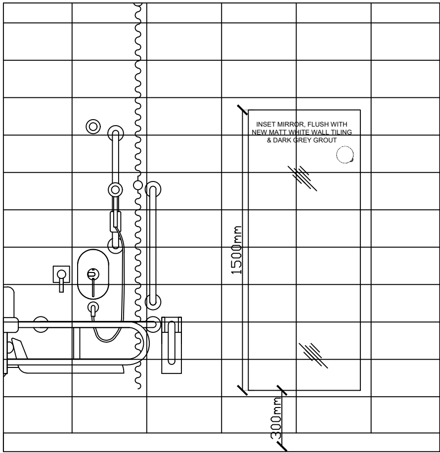
ELEVATION C-C
