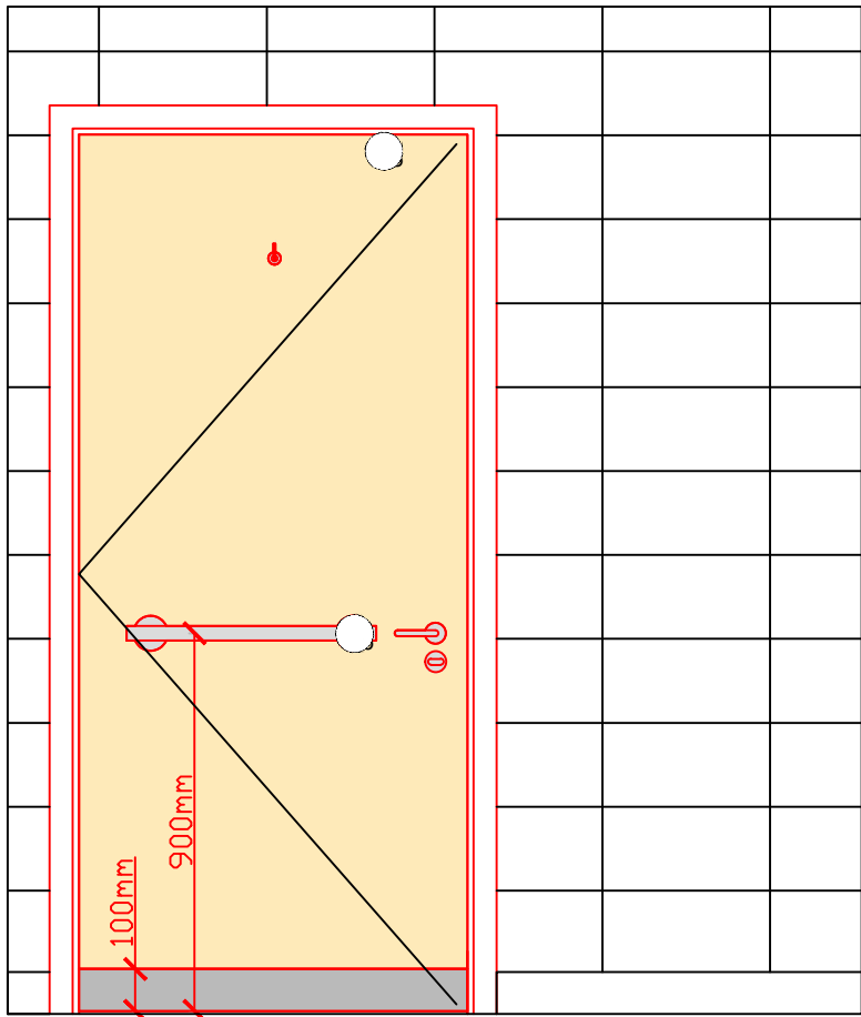
ELEVATION D-D
