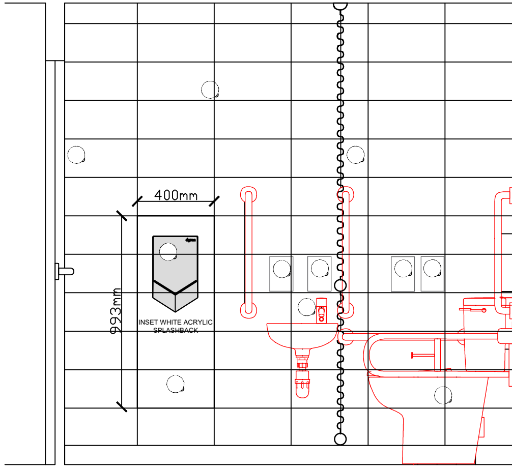
ELEVATION A-A
