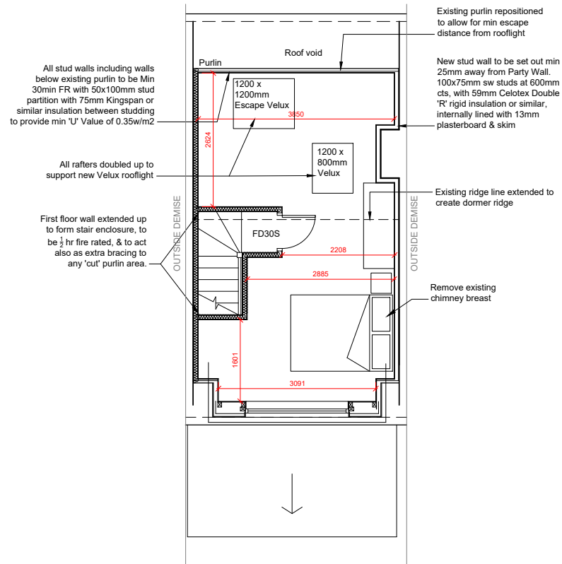
LOFT PLAN
