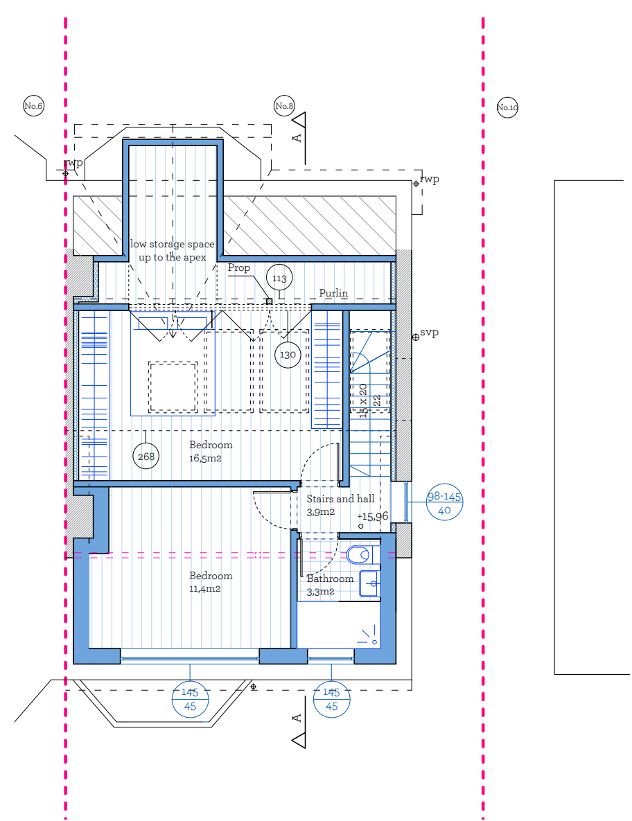
Loft Plan
