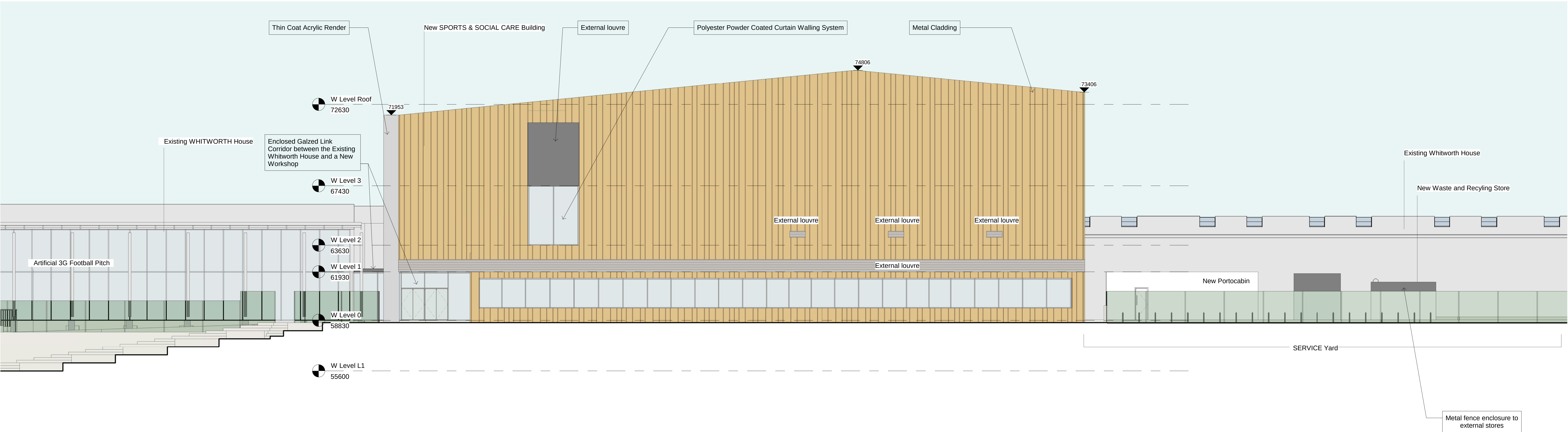
2 West 1-100 1 : 100
