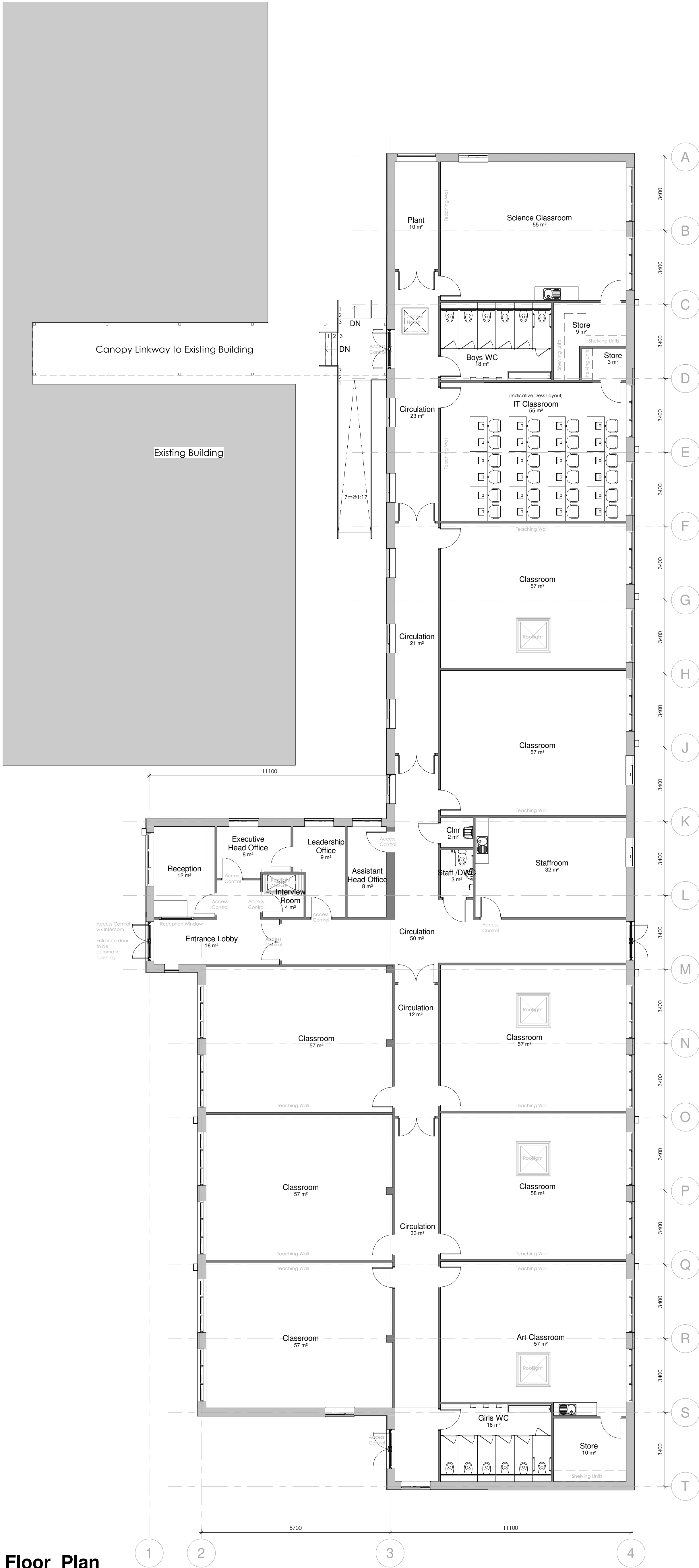
00_Ground_Floor_Plan 1 : 100
