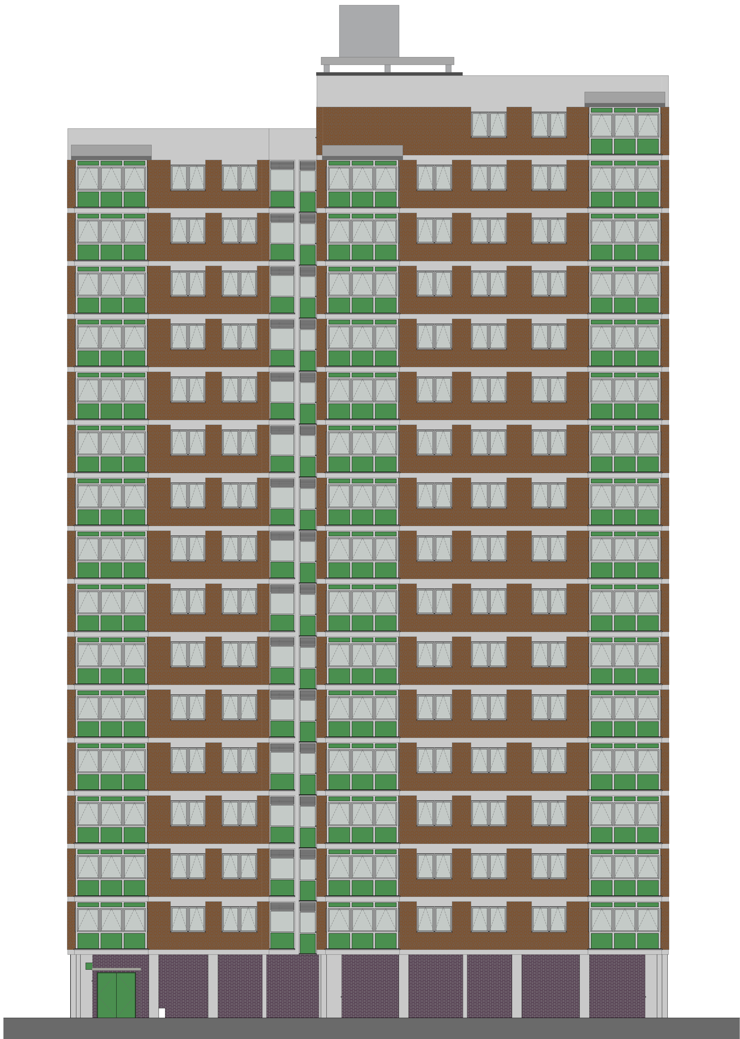
2 Elevation 1:100
