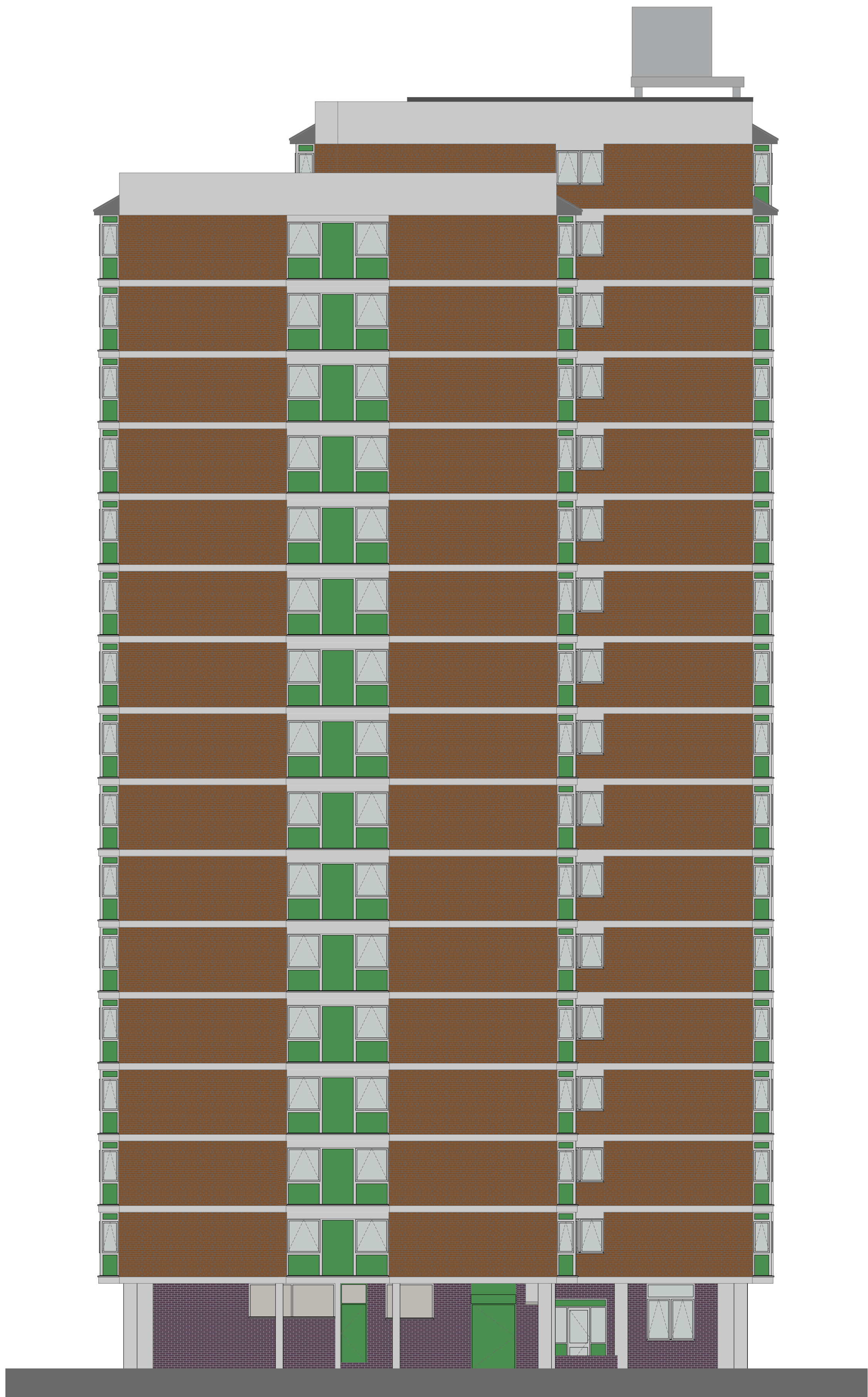
1 Elevation 1:100
