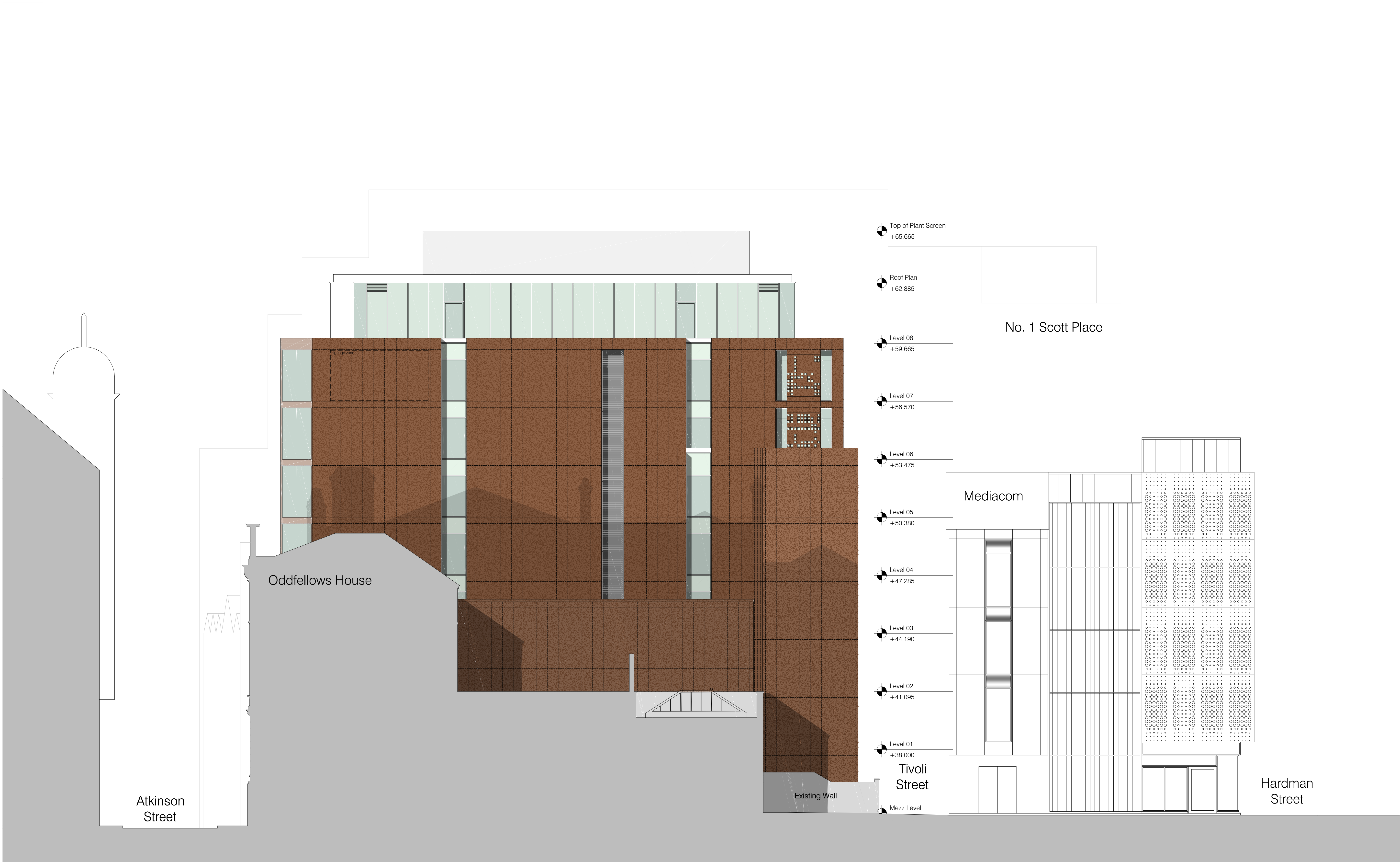
Deansgate Elevation Scale: 1:100
