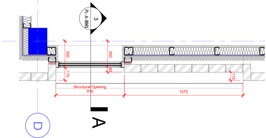
2 Plan Extract 1 : 25
