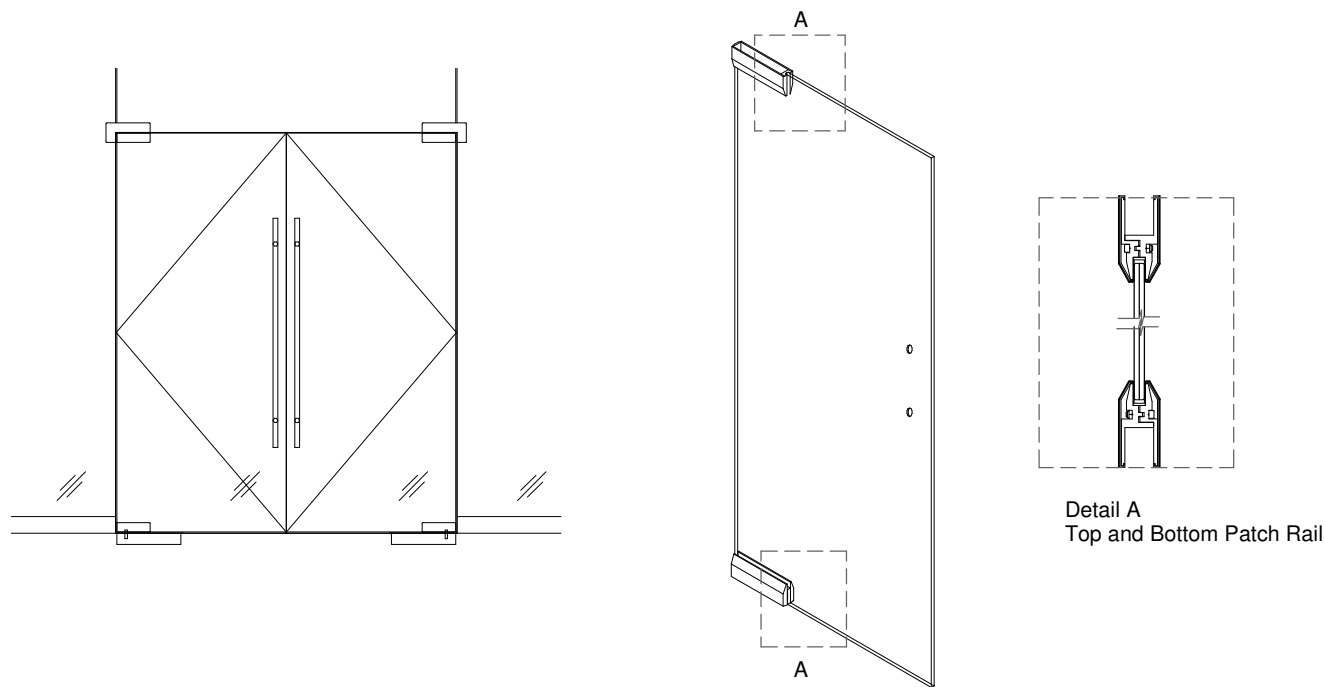
3 Detail Frameless Door NTS
