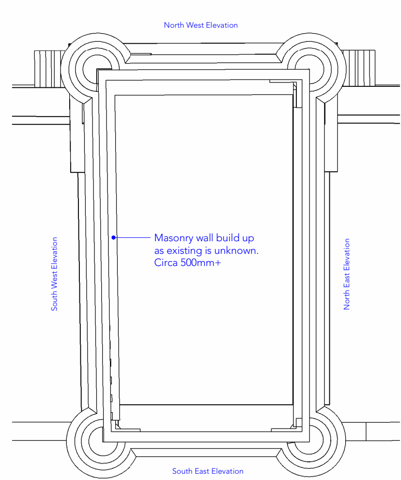
9 Tower Plan 1 : 50
