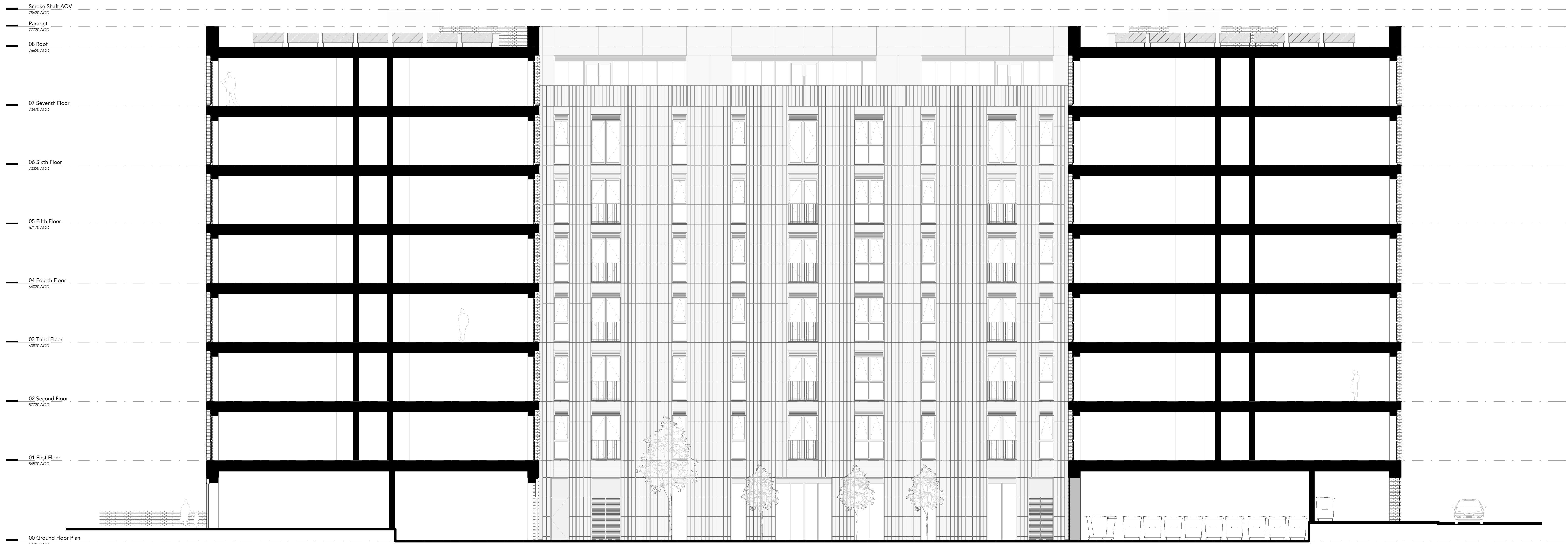
Section 1-1 1:100
