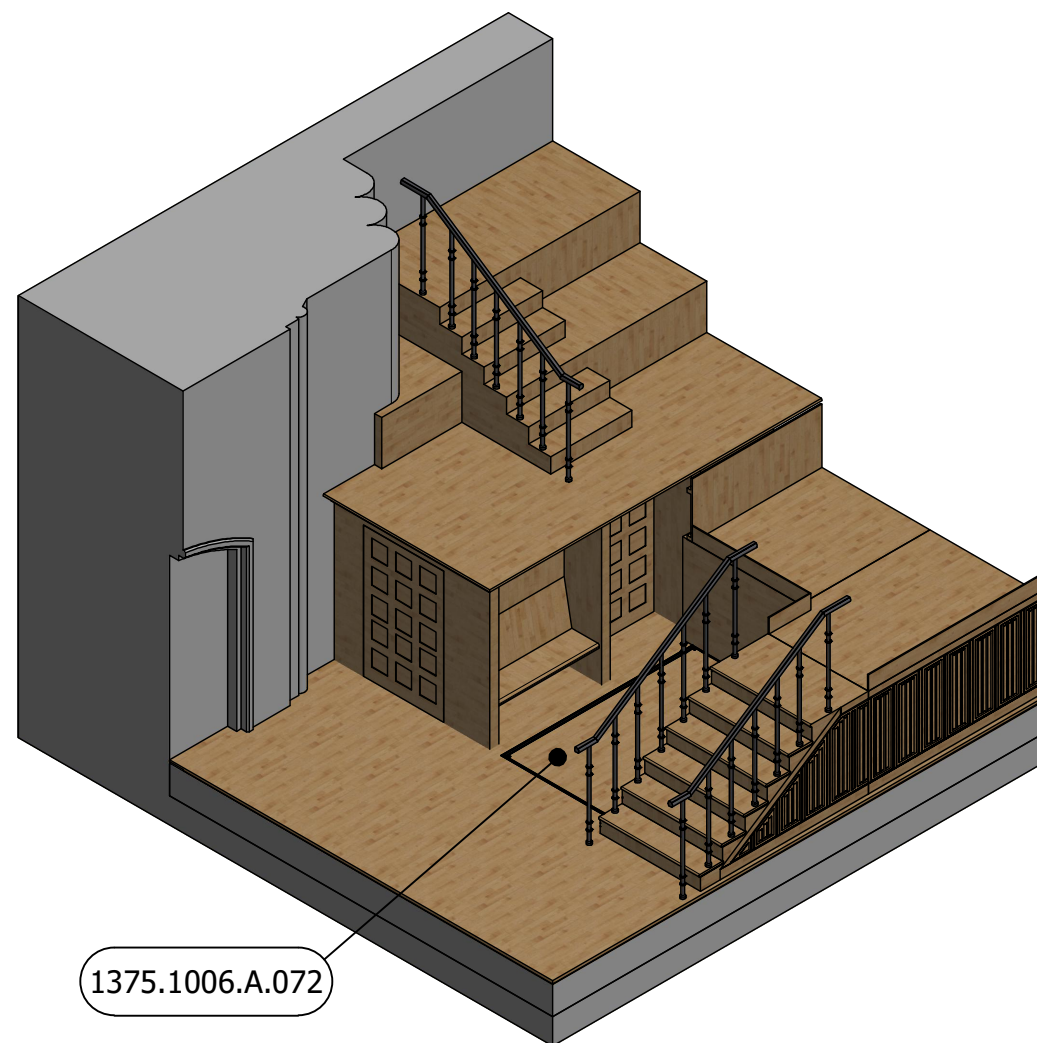
A-A ( 1 : 30 )
