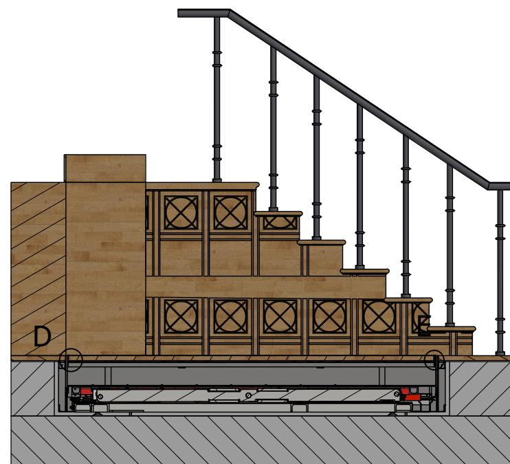
A-A ( 1 : 30 )
