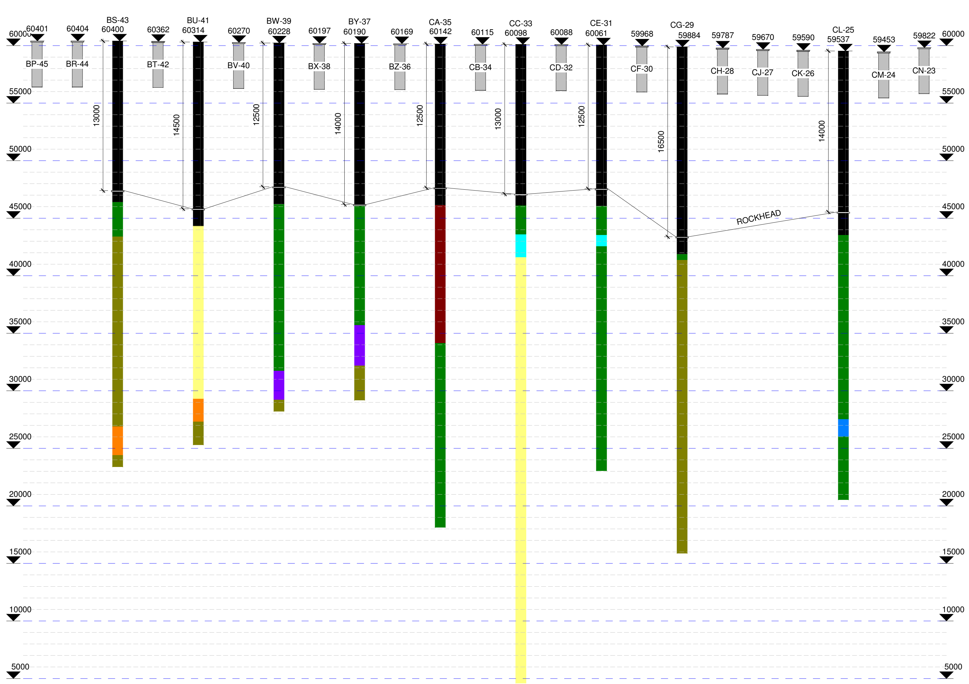
Section 5 1 : 200
