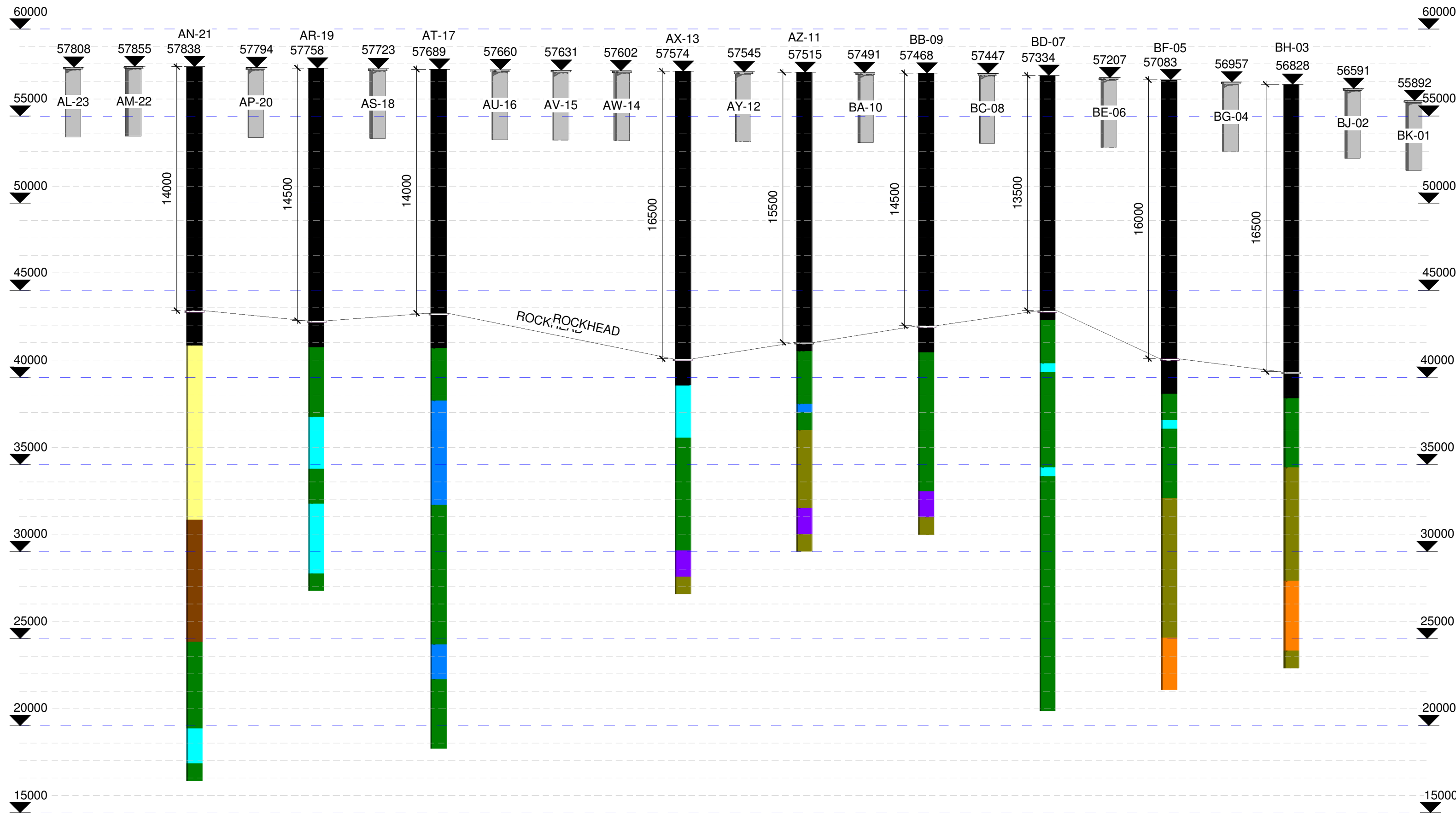
Section 1 1 : 200
