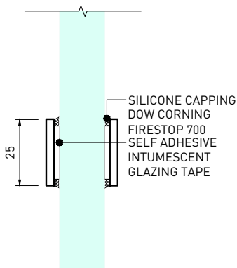
06 LOFT BARS SCALE 1:2
