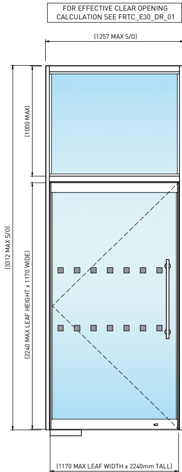
02 SINGLE DOOR MAX WIDTH SCALE 1:35
