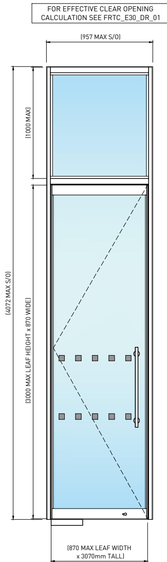
01 SINGLE DOOR MAX HEIGHT SCALE 1:35
