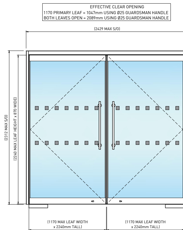
02 DOUBLE DOORSET - MAX WIDTH SCALE 1:35
