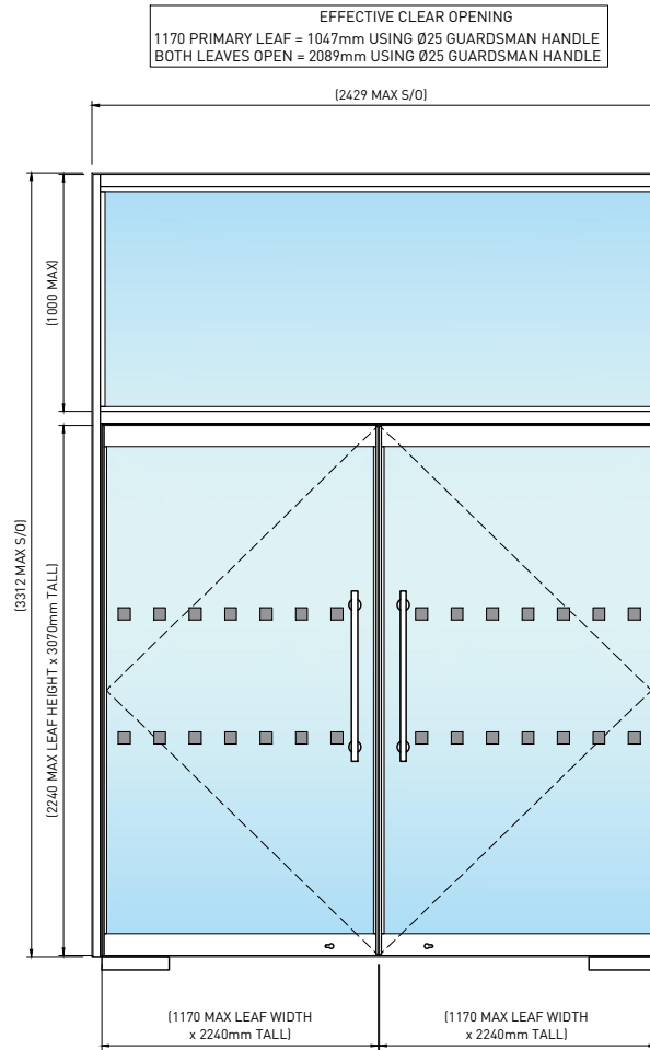
02 DOUBLE DOORSET - MAX WIDTH SCALE 1:35
