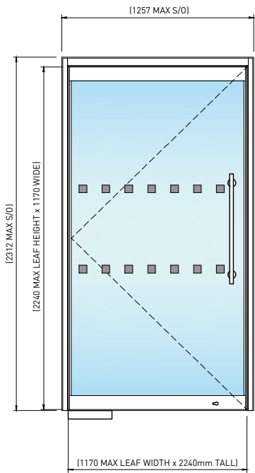
02 SINGLE DOOR MAX WIDTH SCALE 1:35
