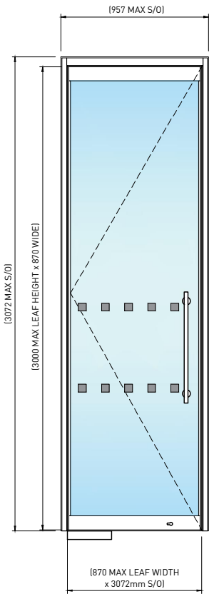
01 SINGLE DOOR MAX HEIGHT SCALE 1:35
