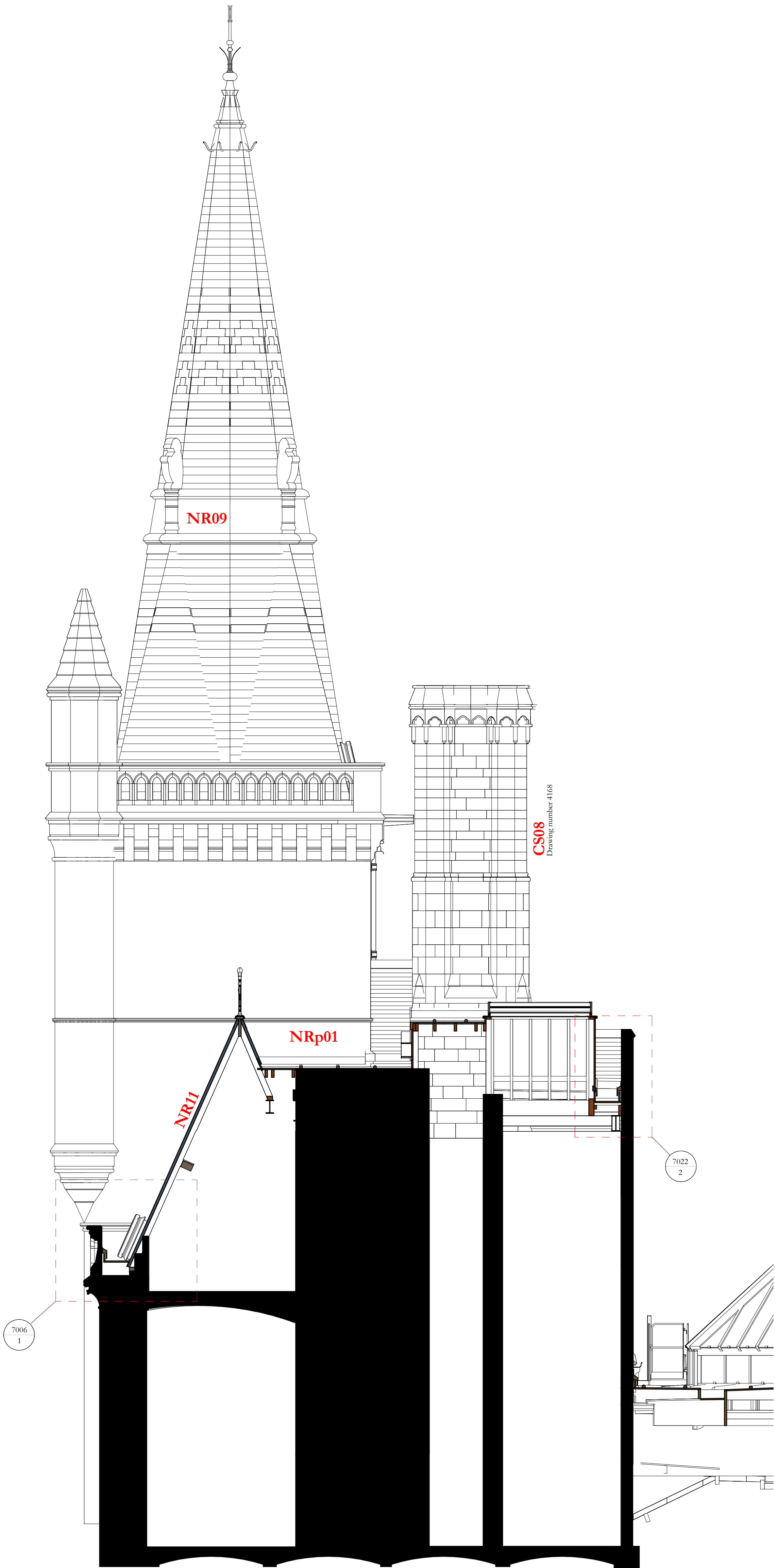
Section PP 1 : 50
