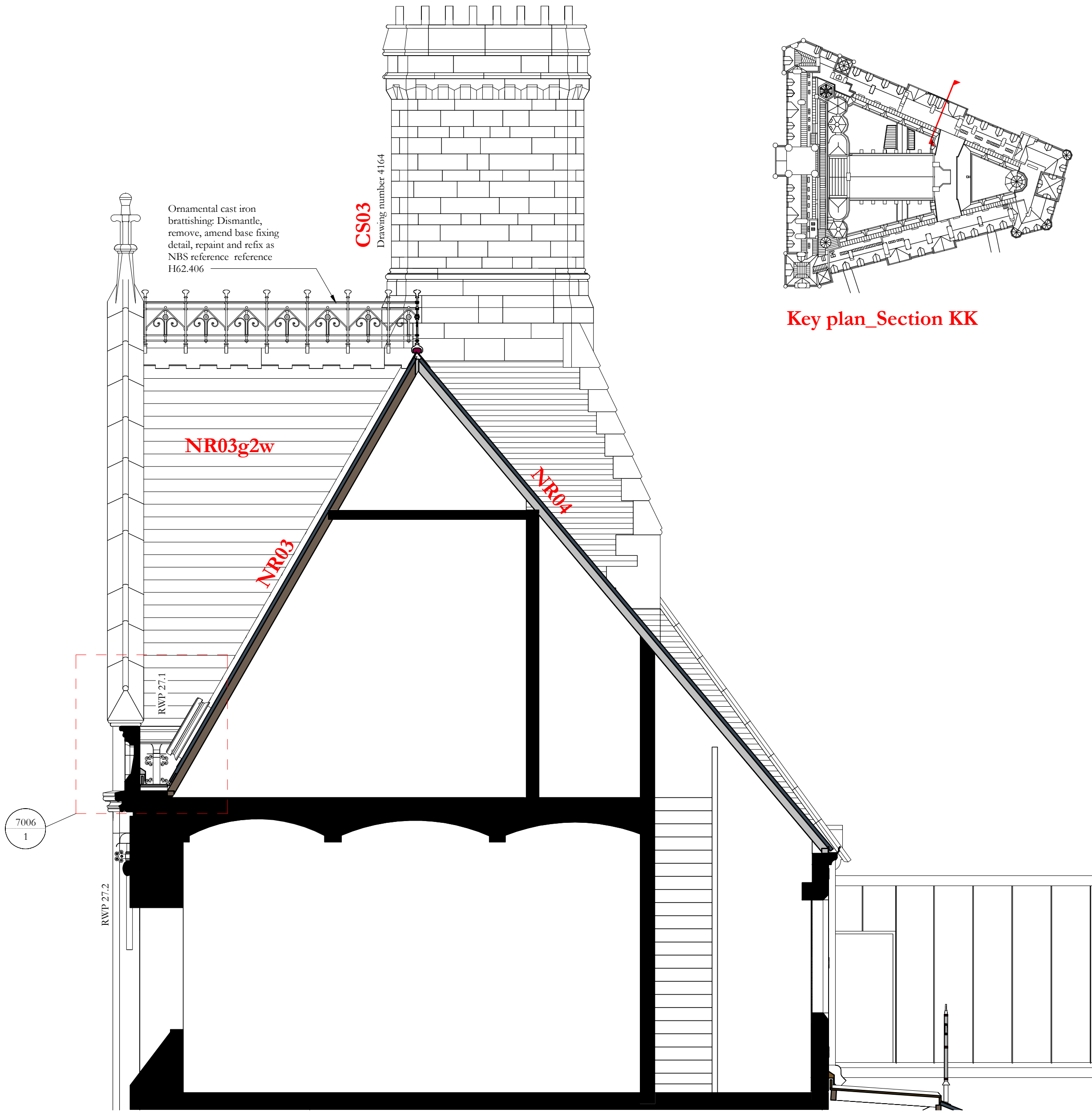
Section KK 1 : 50
