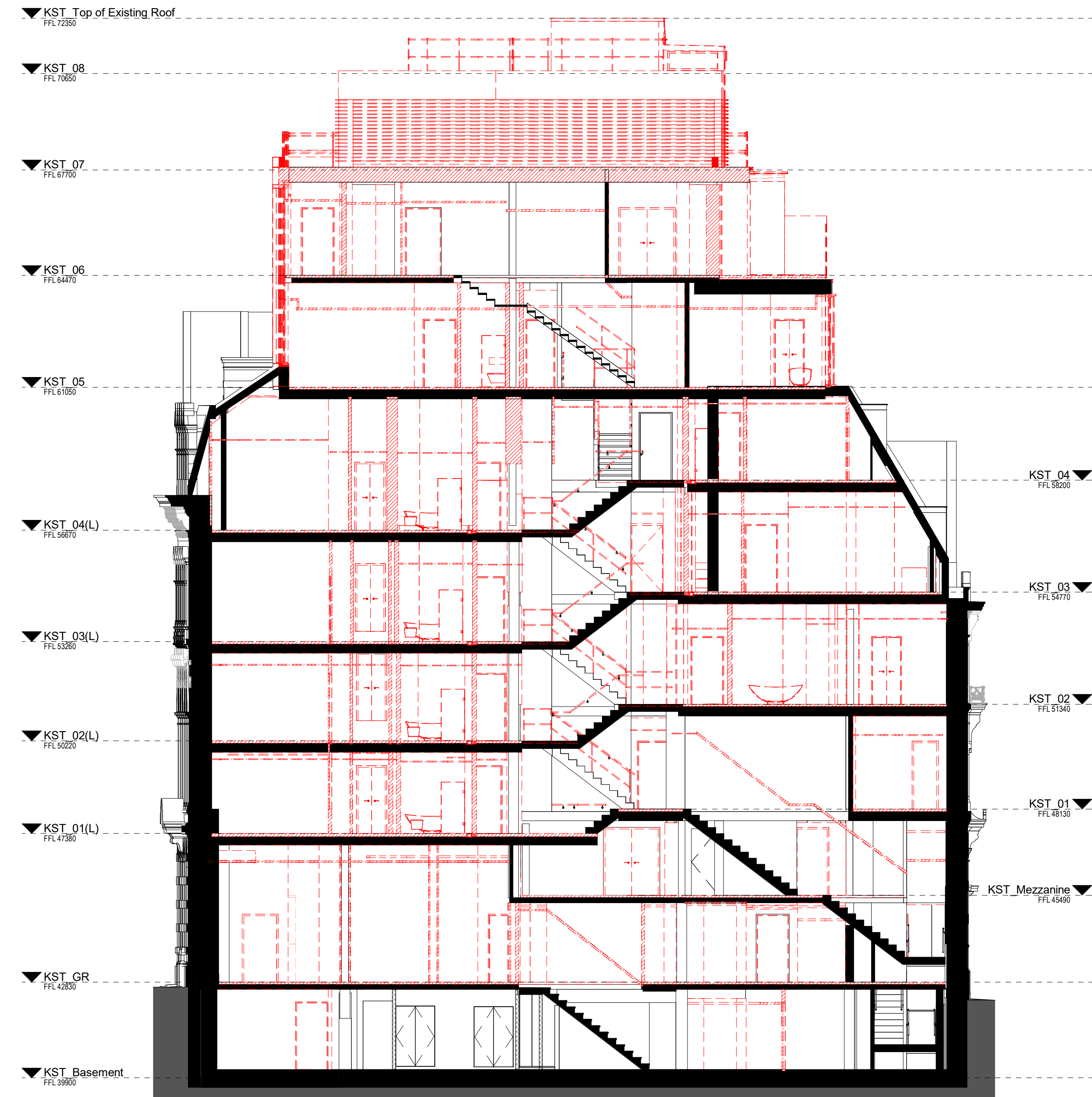
1 Demolition Section AA 1 : 100
