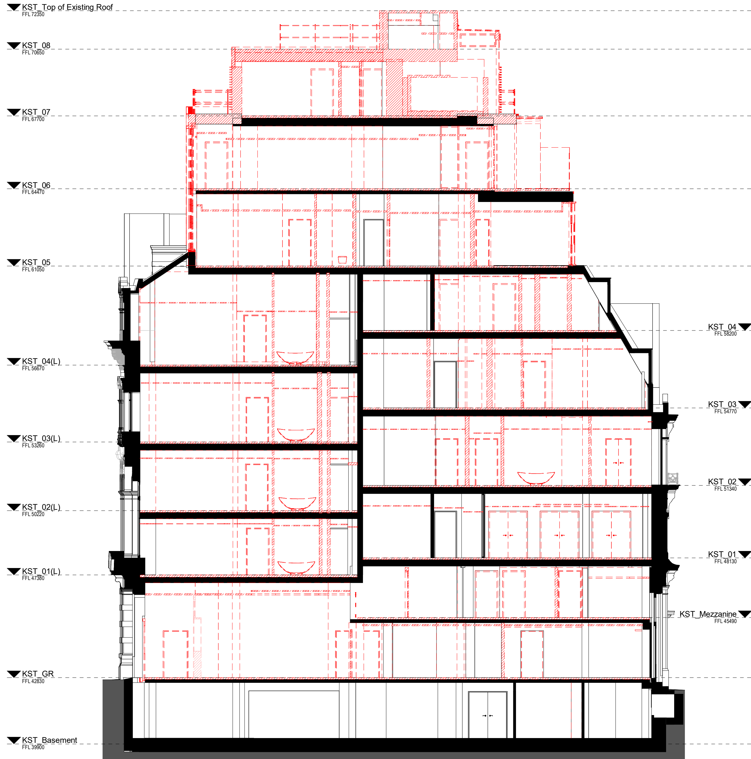
2 Demolition Section BB 1 : 100
