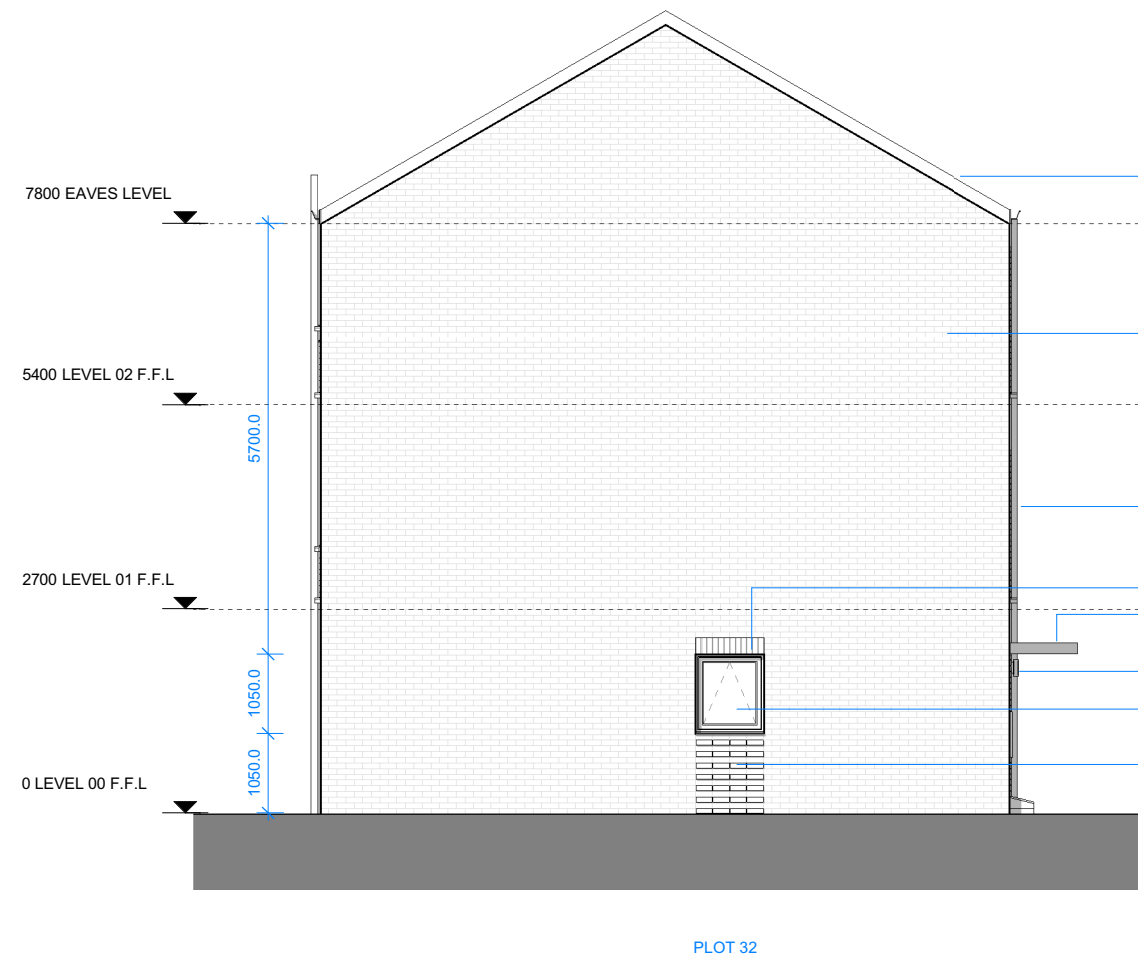
6 | HT D1 - 4B5P M4(1) - SIDE ELEVATION 01 1:100
