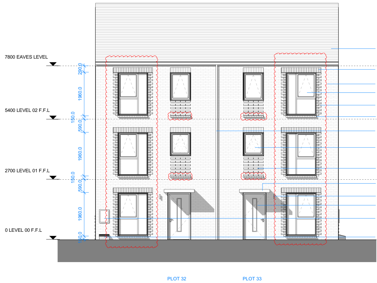
5 | HT D1 - 4B5P M4(1) - FRONT ELEVATION 1:100
