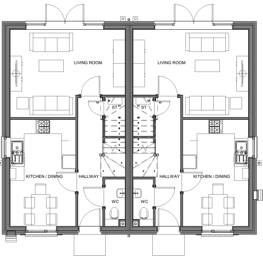
1 | HT D1 - 4B5P M4(1) - 00 PLAN 1:100
