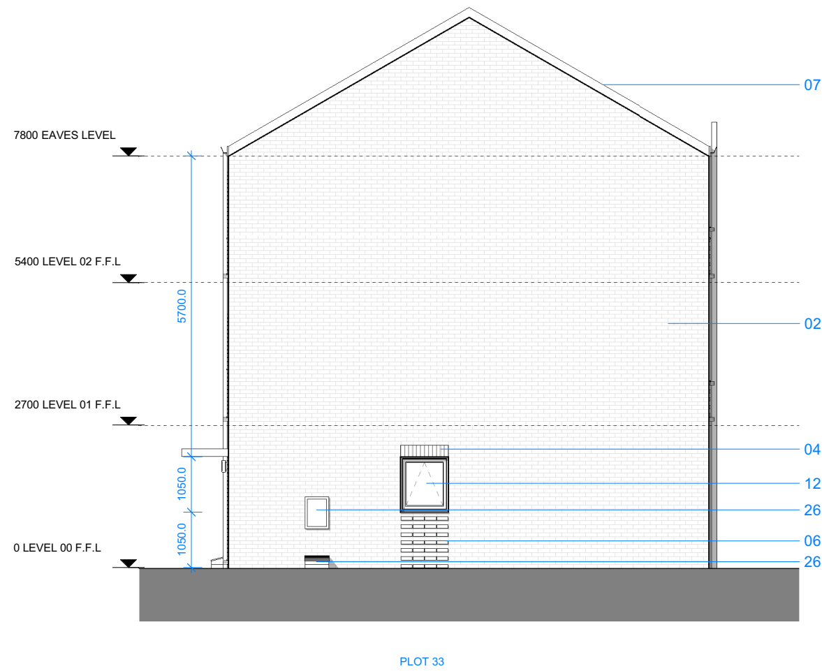
8 | HT D1 - 4B5P M4(1) - SIDE ELEVATION 02 1:100
