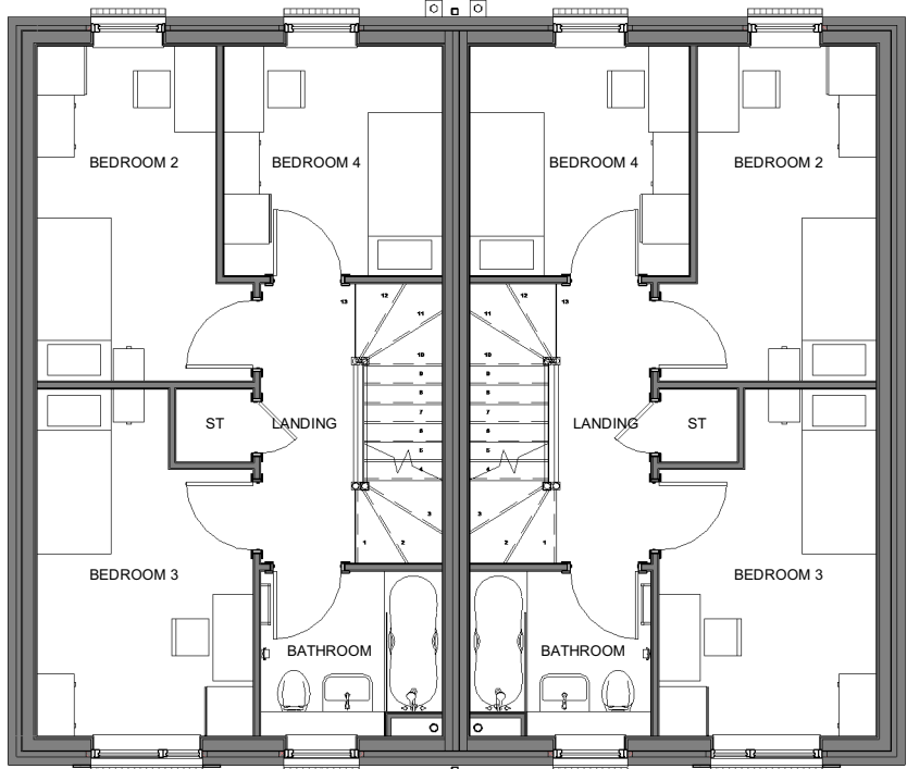
2 | HT D1 - 4B5P M4(1) - 01 PLAN 1:100
