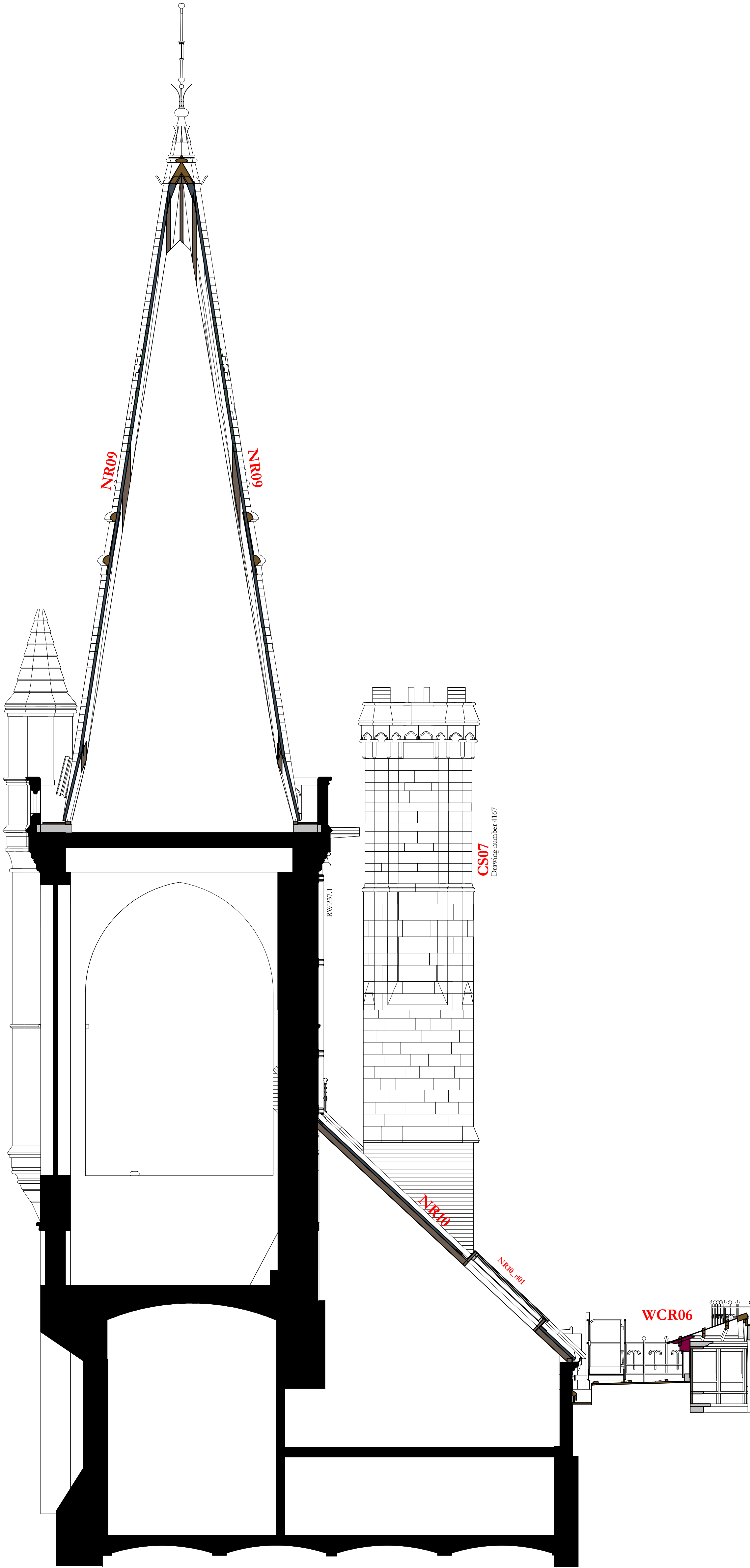
Section OO 1 : 50
