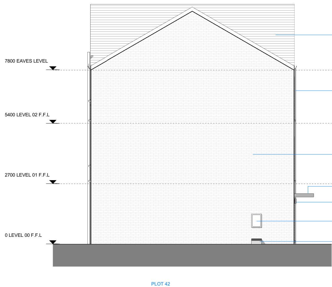
6 | HT D4 - 4B5P M4(1) - SIDE ELEVATION 01 1 : 100
