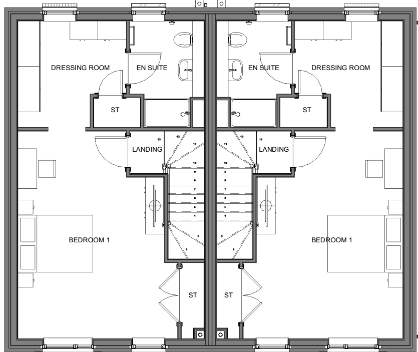
3 | HT D4 - 4B5P M4(1) - 02 PLAN 1 : 100
