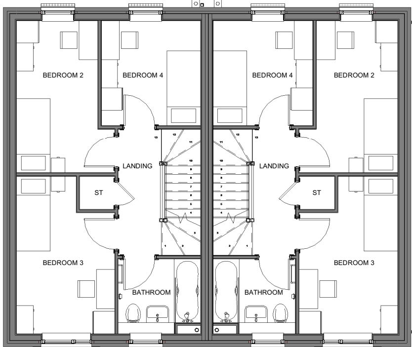
2 | HT D4 - 4B5P M4(1) - 01 PLAN 1 : 100
