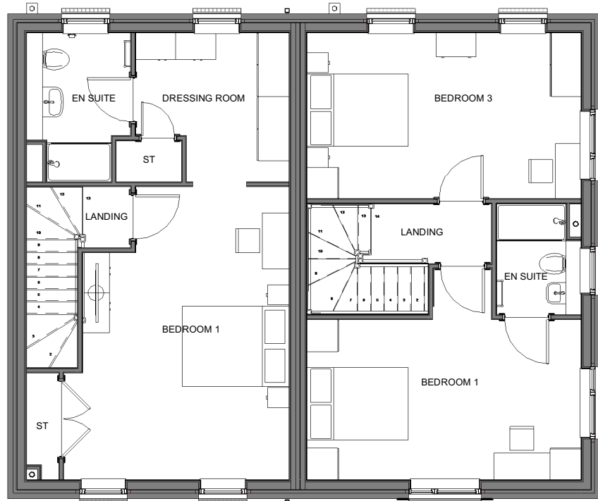
3 | HT D2 - 4B5P & 4B7P M4(1) - 02 PLAN 1 : 100
