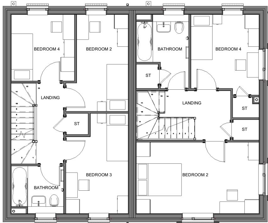
2 | HT D2 - 4B5P & 4B7P M4(1) - 01 PLAN 1 : 100
