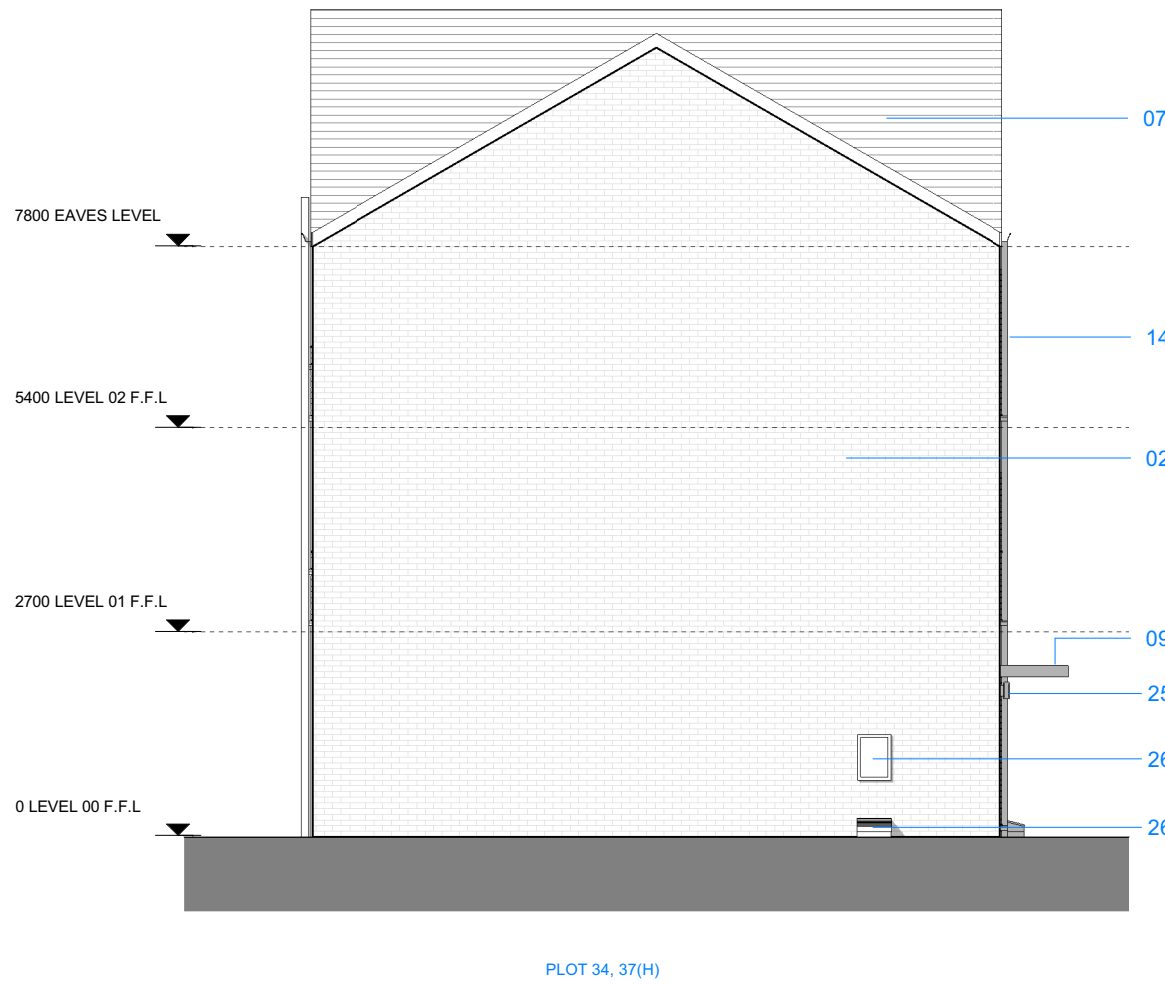
6 | HT D2 - 4B5P & 4B7P M4(1) - SIDE ELEVATION 01 1 : 100
