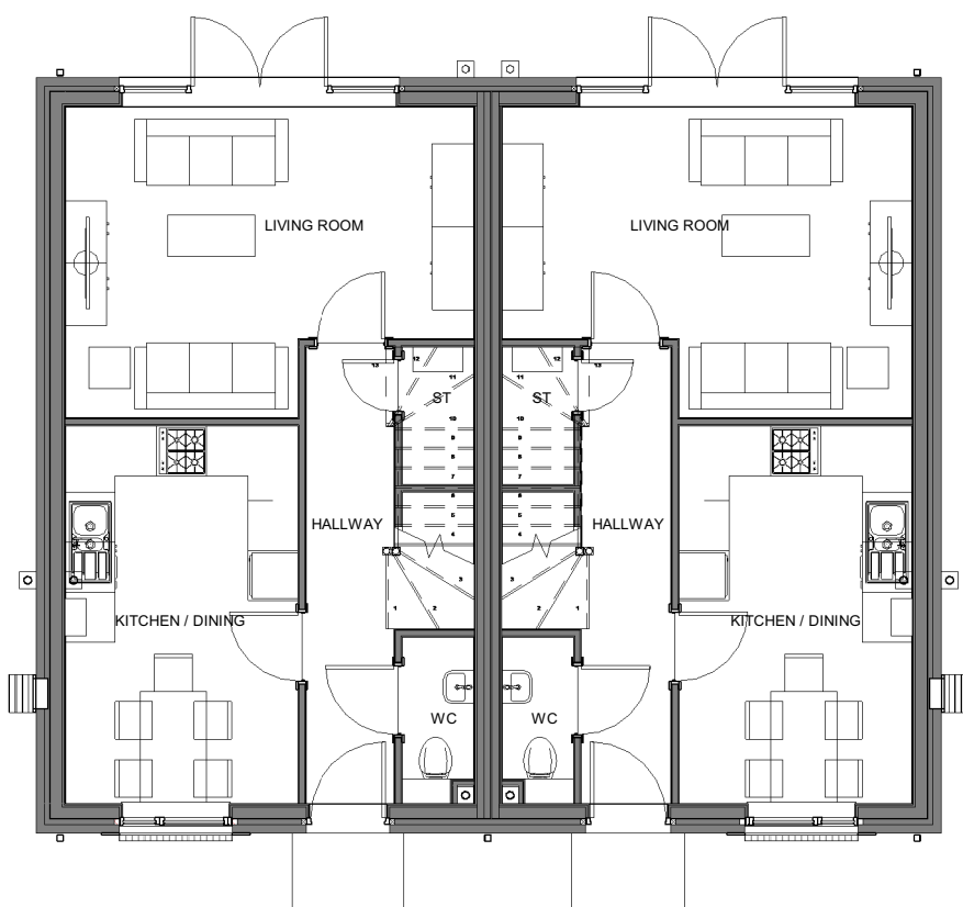
1 | HT D3 - 4B5P M4(1) - 00 PLAN 1 : 100
