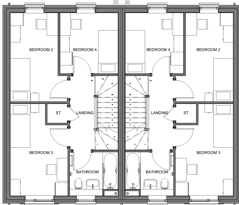
2 | HT D3 - 4B5P M4(1) - 01 PLAN 1 : 100
