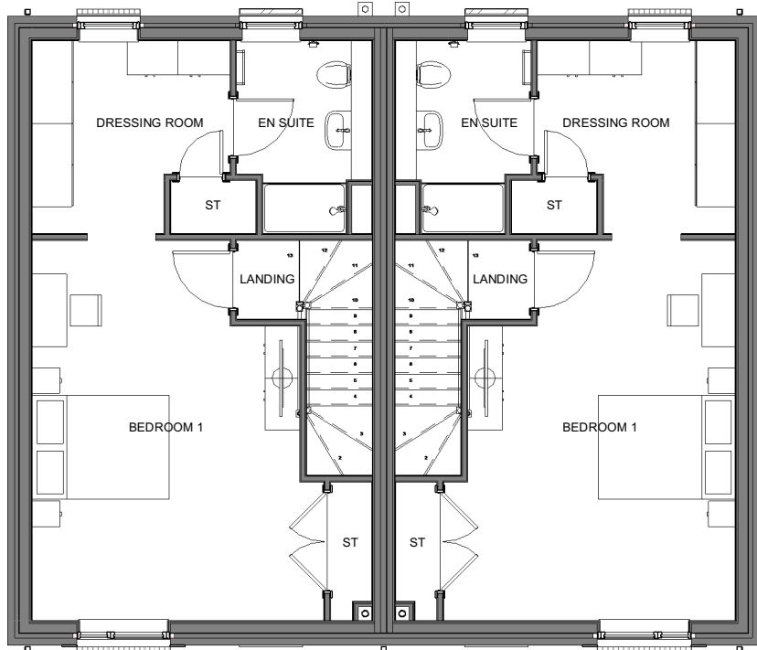
3 | HT D3 - 4B5P M4(1) - 02 PLAN 1 : 100
