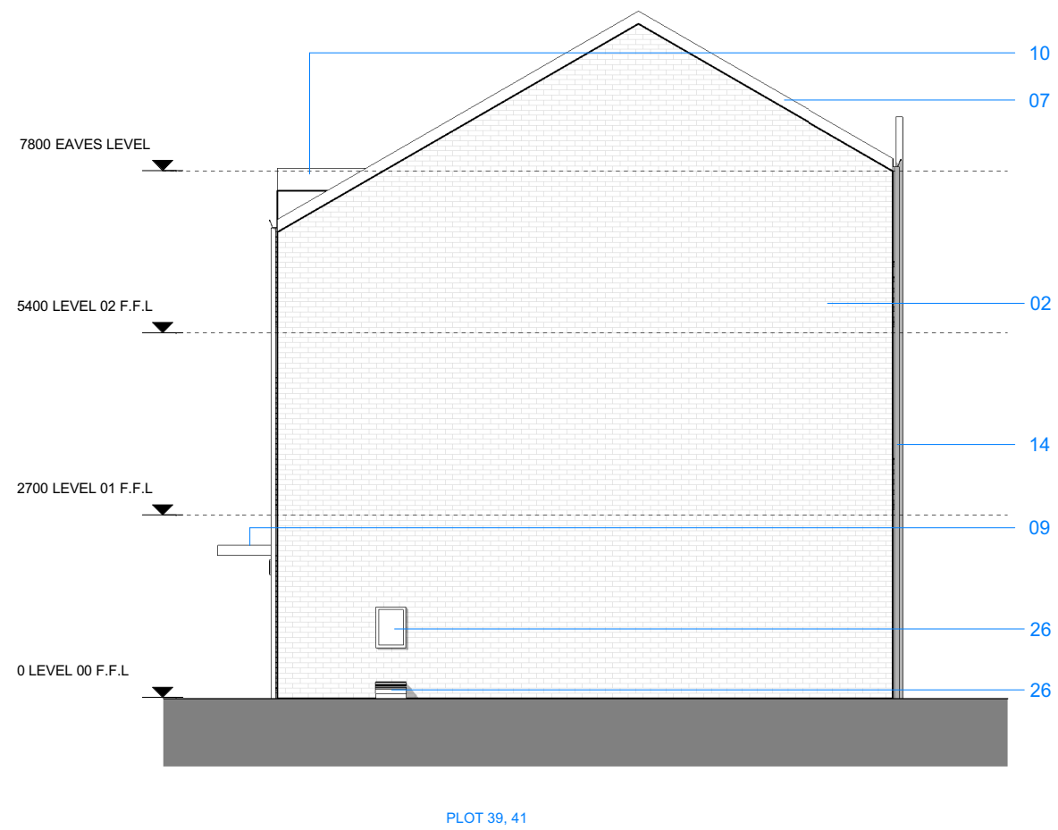
8 | HT D3 - 4B5P M4(1) - SIDE ELEVATION 02 1 : 100
