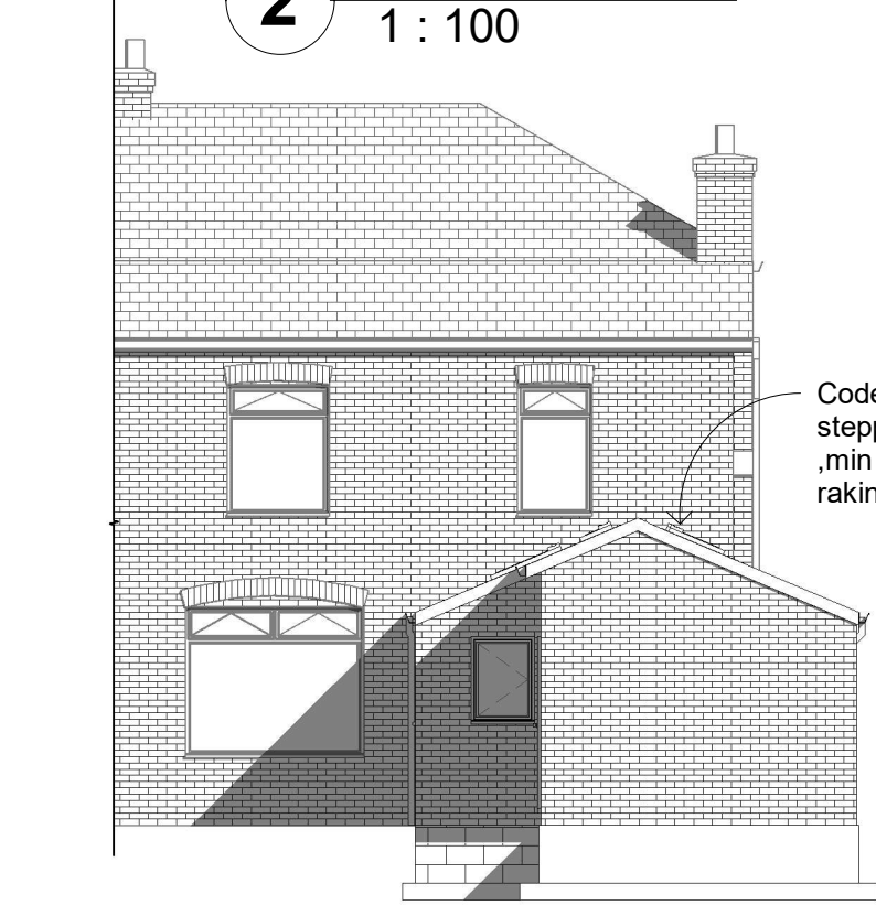
3 Rear 1 : 100
