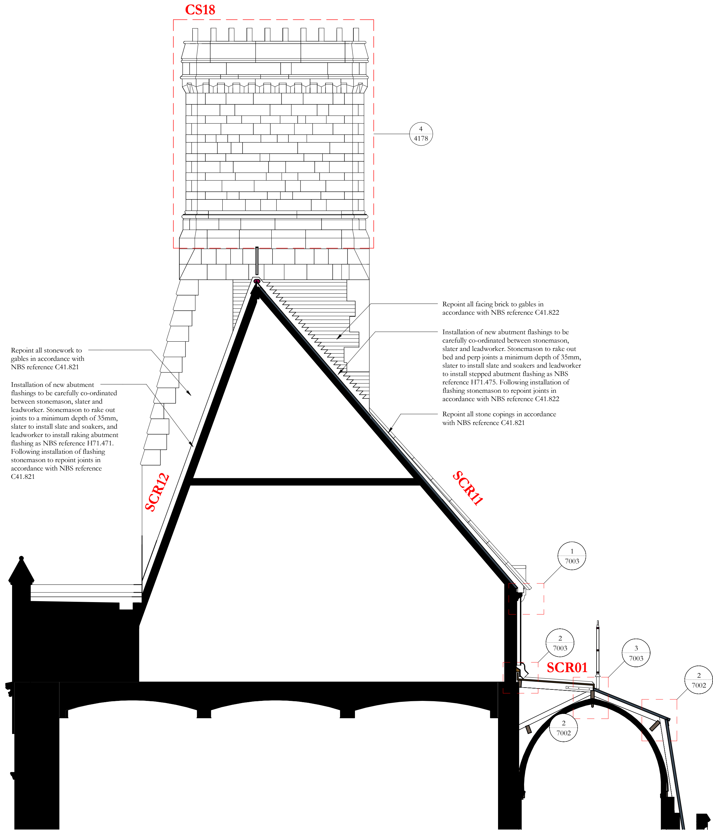
Section AX 1 : 50
