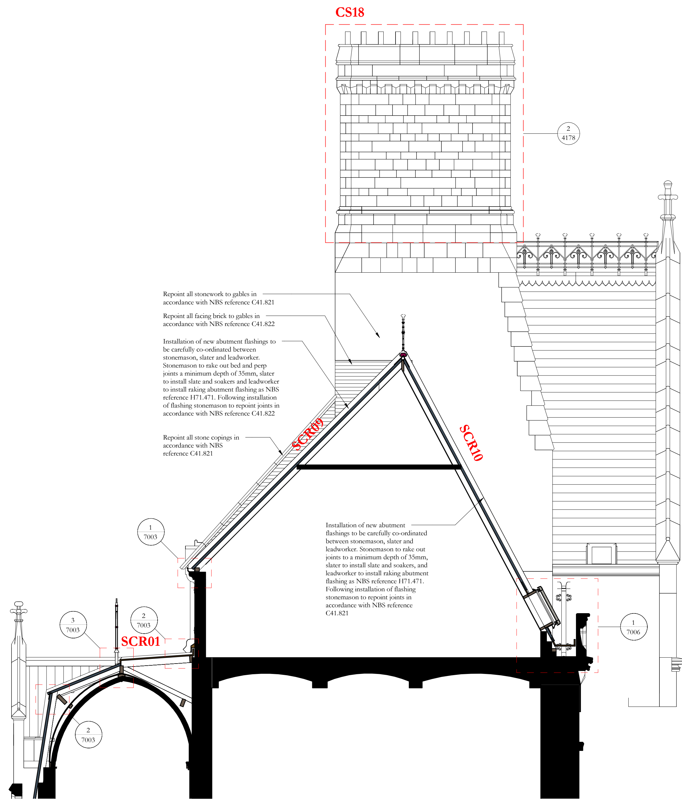
Section AW 1 : 50
