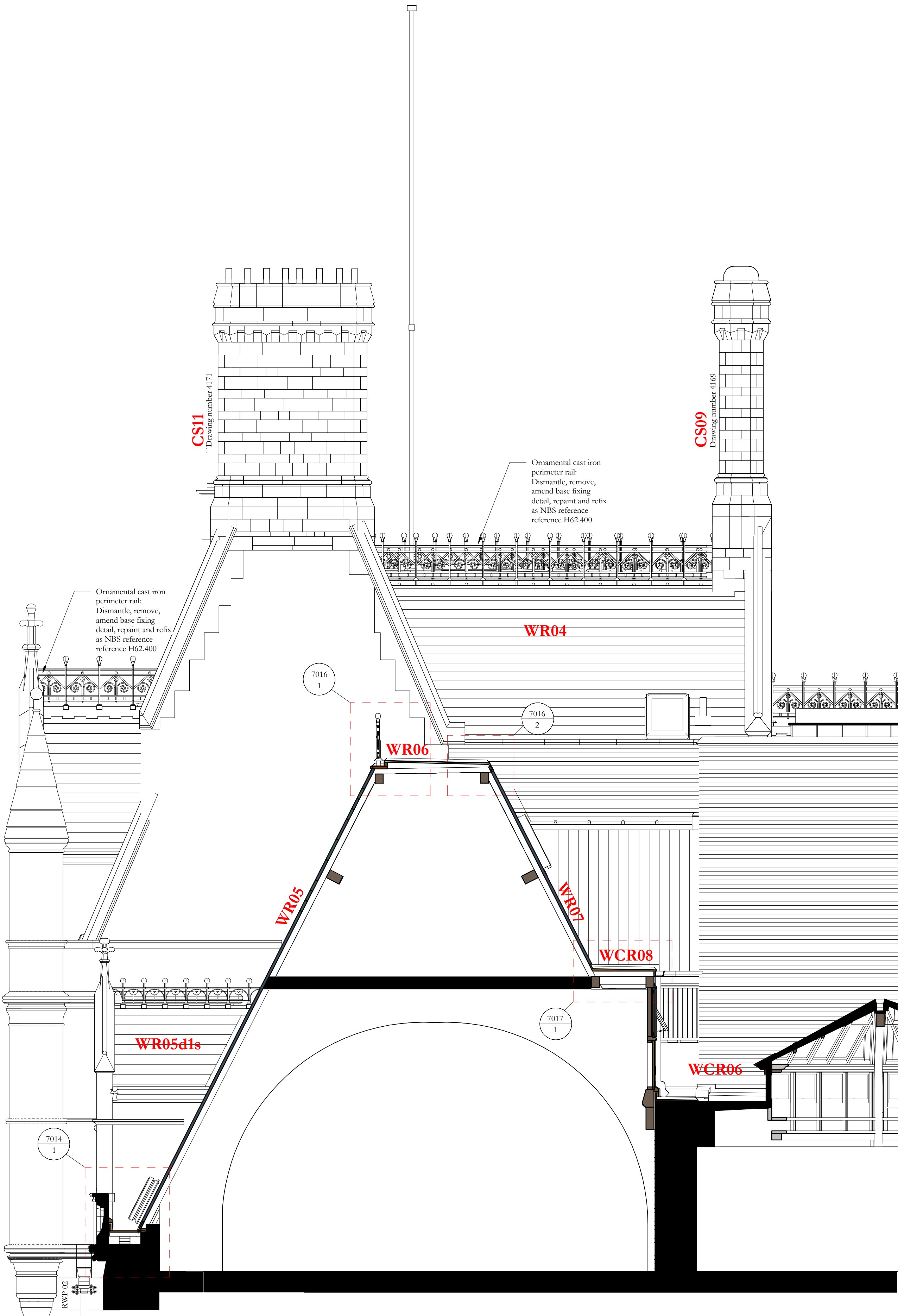
Section SS 1 : 50
