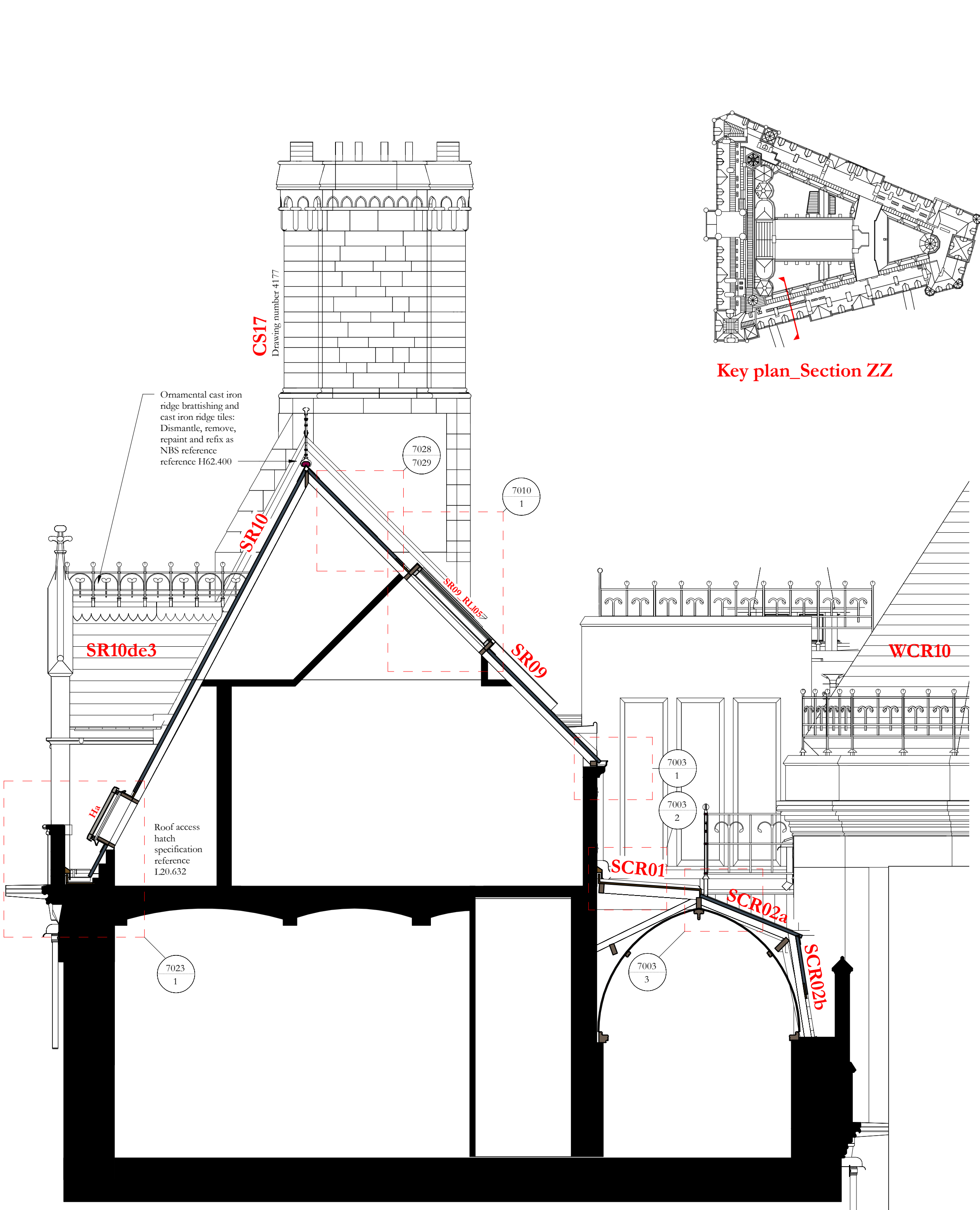
Section ZZ 1 : 50
