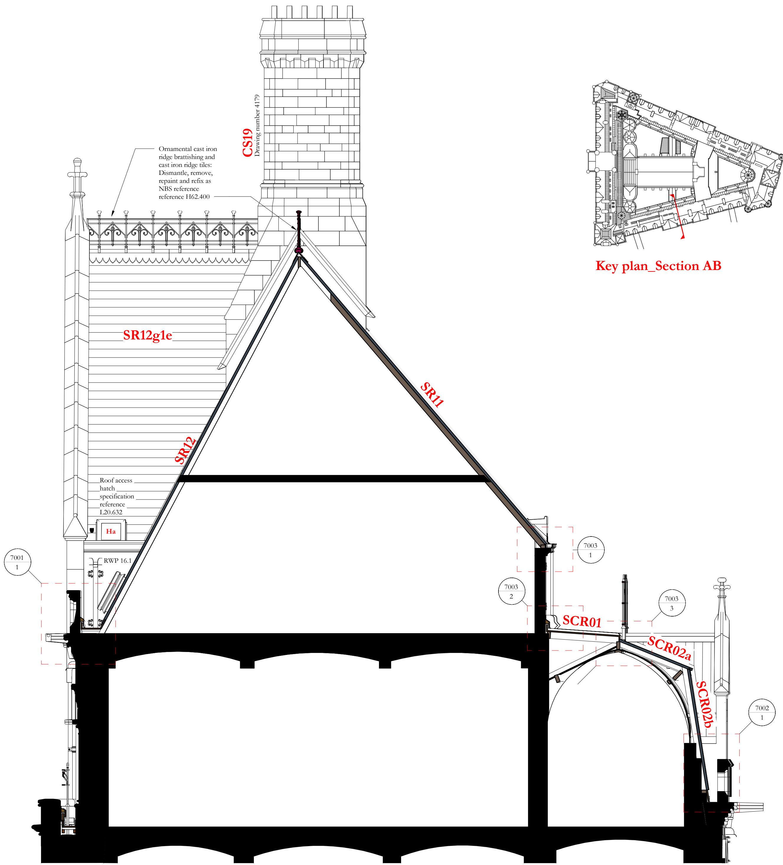
Section AB 1 : 50
