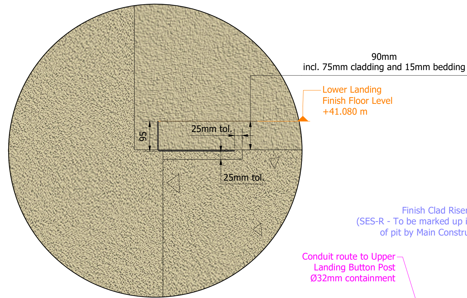
AM ( 1 : 7 )
