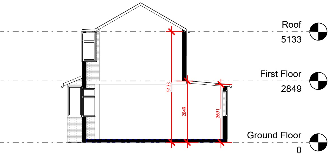
1 Section 1-1 Existing 1 : 100
