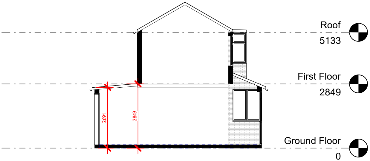
2 Section 2-2 Existing 1 : 100
