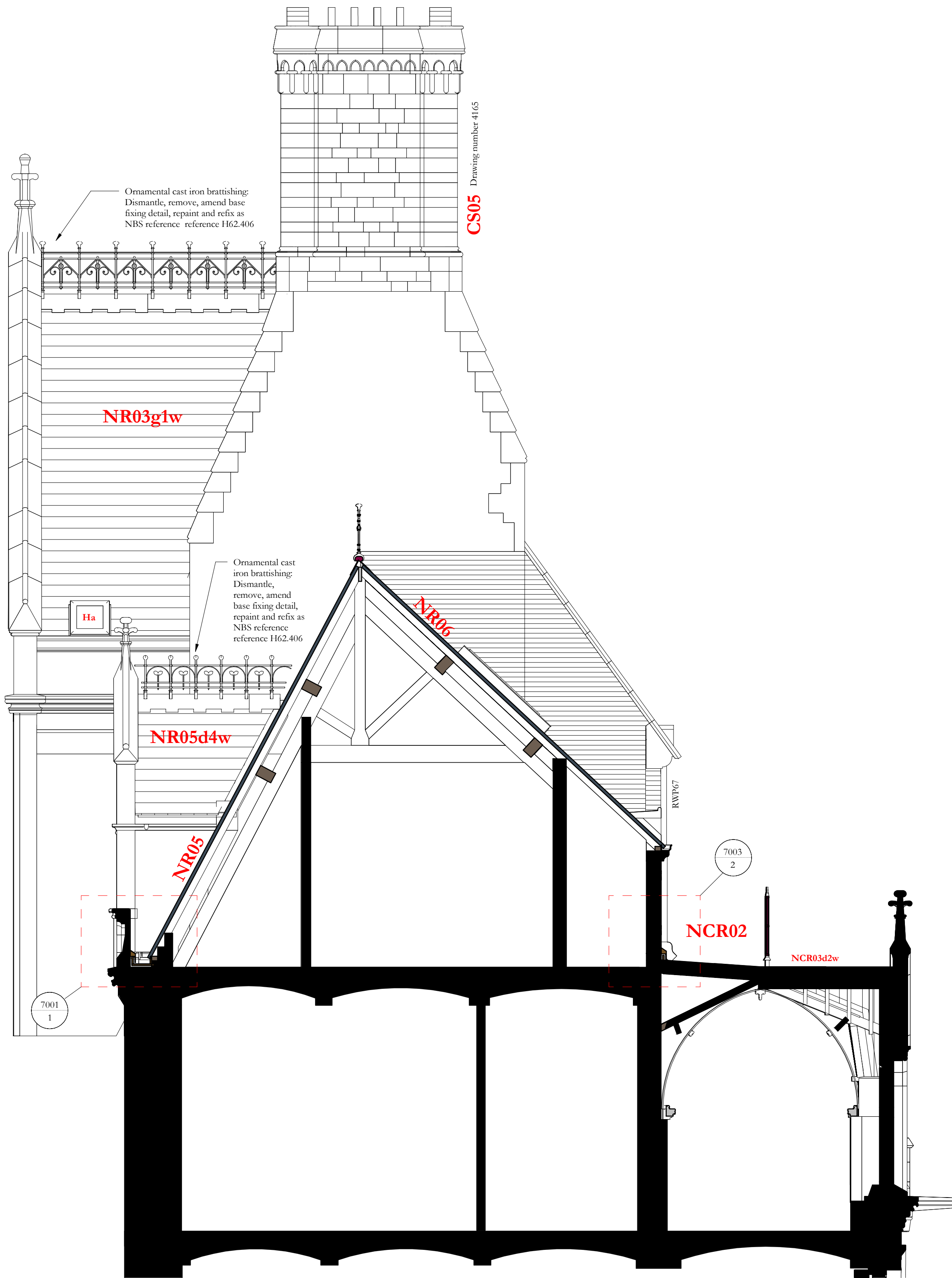
Section MM 1 : 50
