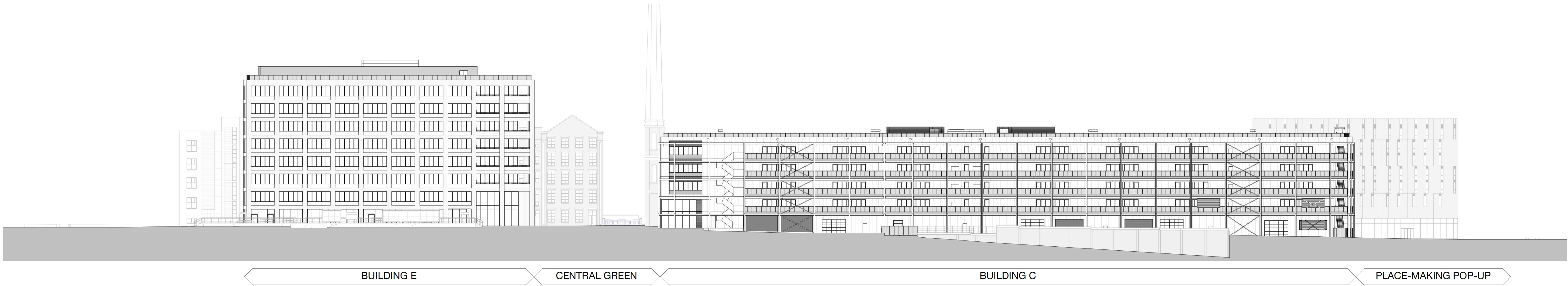
Long Site Elevation C 1 : 500
