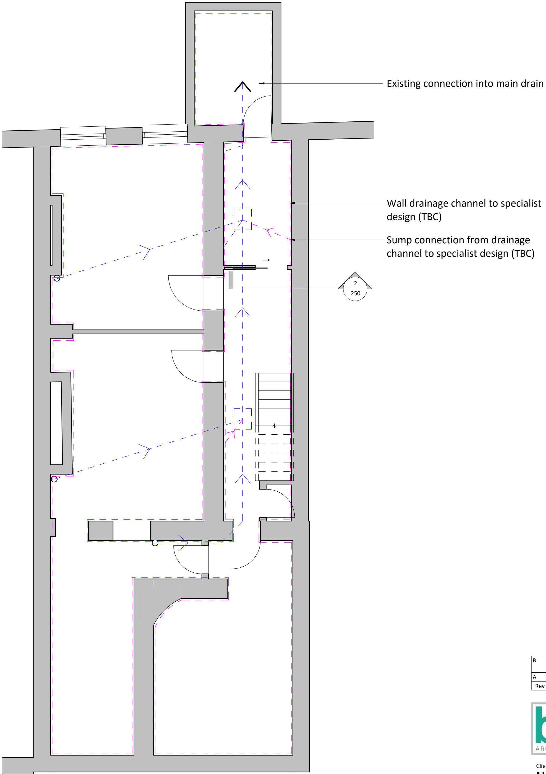
Basement Plan 1 : 50
