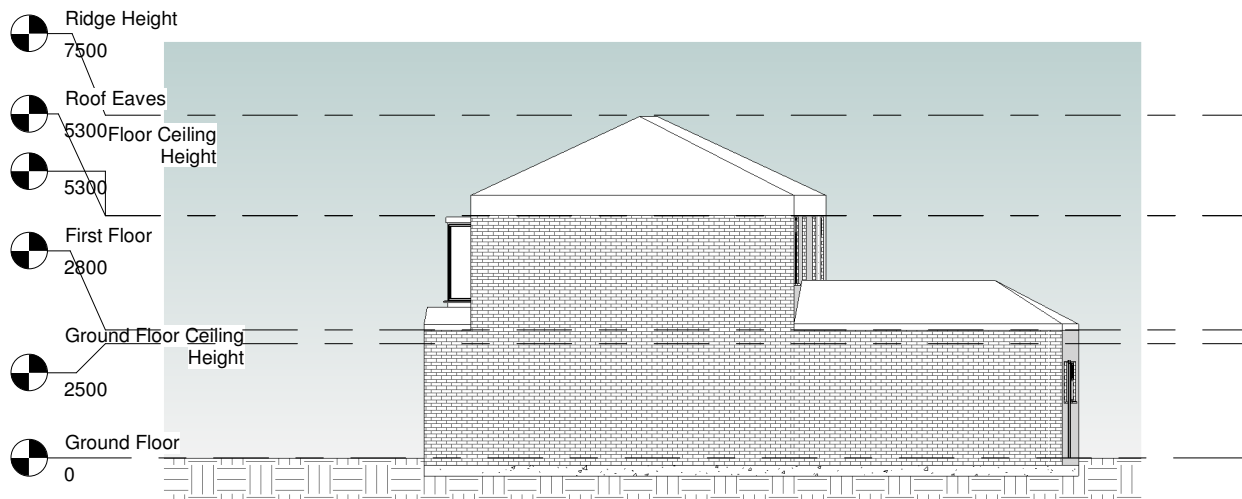
2 West 1 : 100
