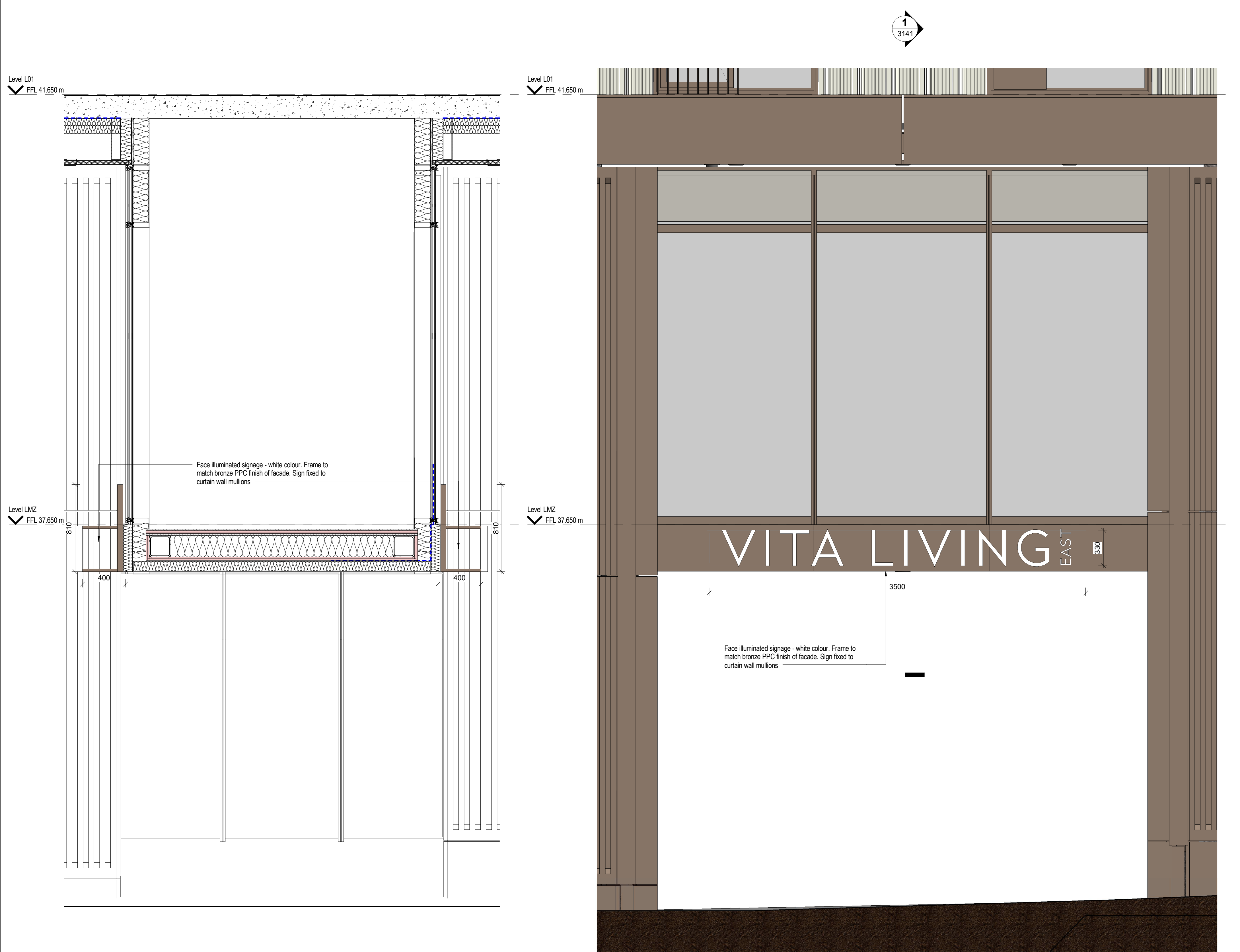
1 Section - GF Signage 1 : 20
