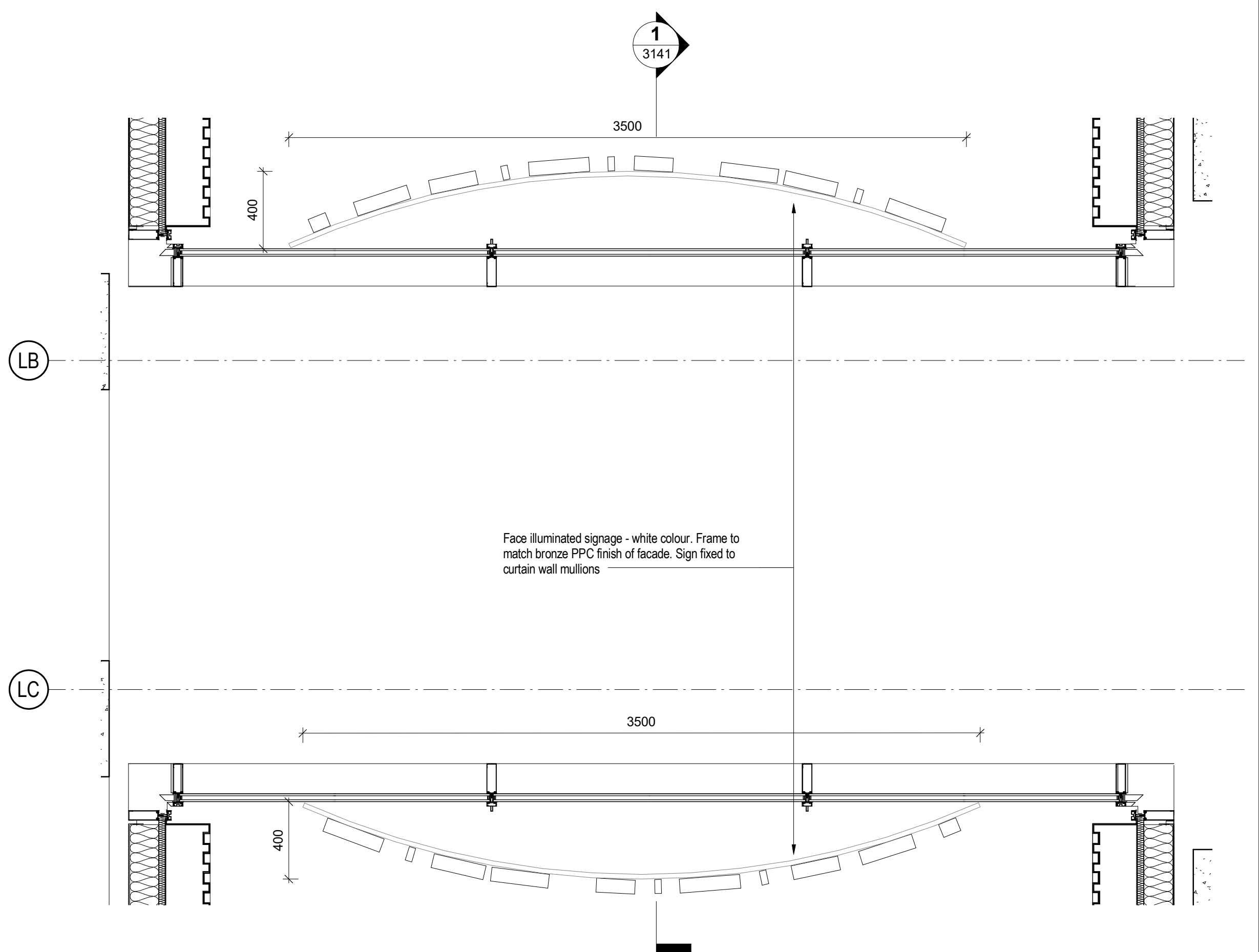
3 Plan - GF Signage 1 : 20
