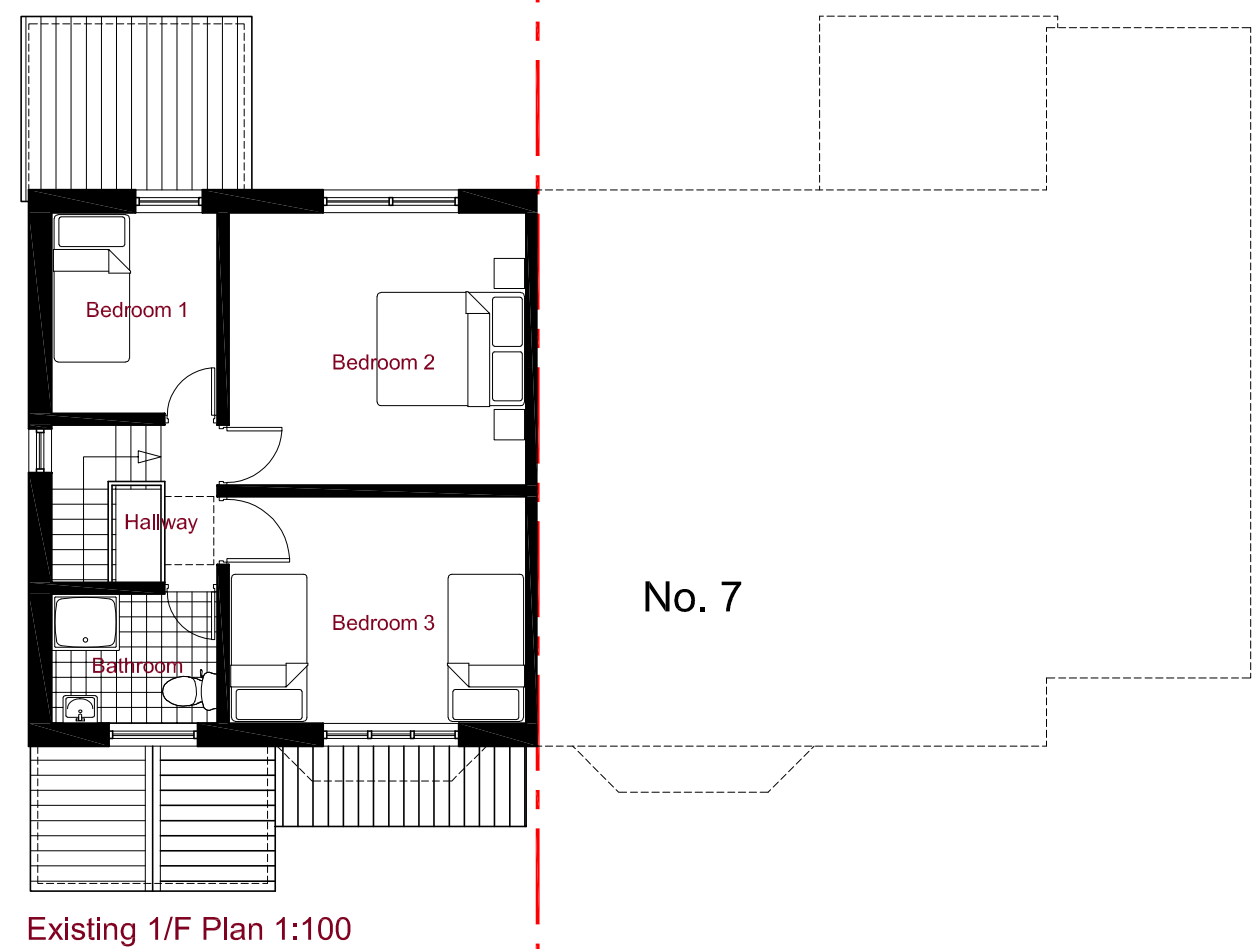
Existing 1/F Plan 1:100
