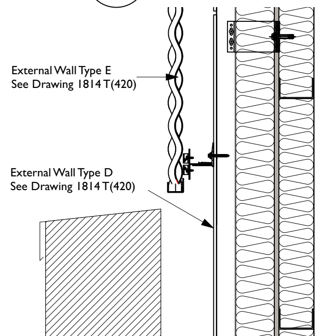
Stair B over Hotel Scale: 1:10
