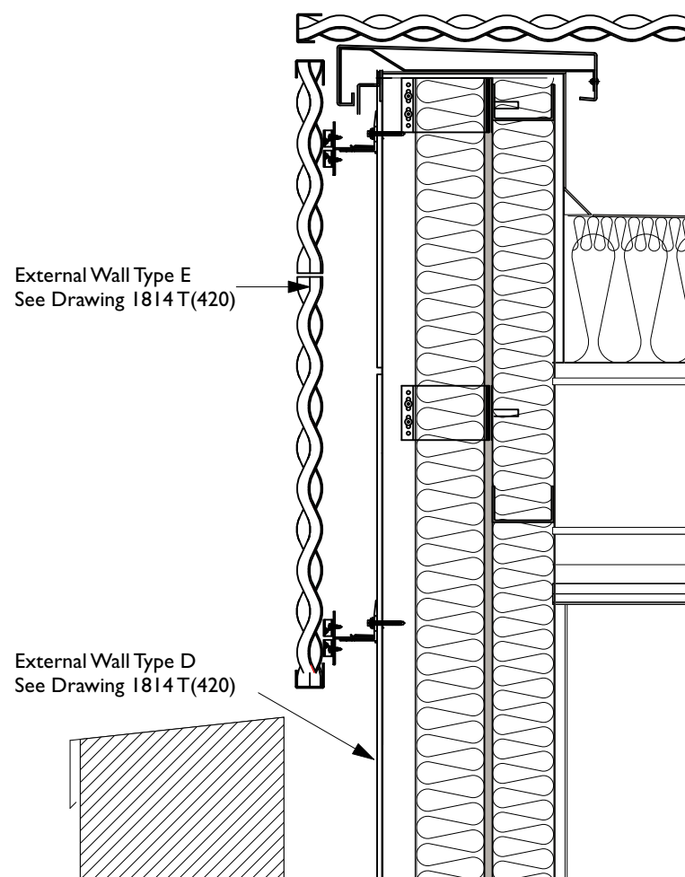
Stair B over Hotel Scale: 1:10
